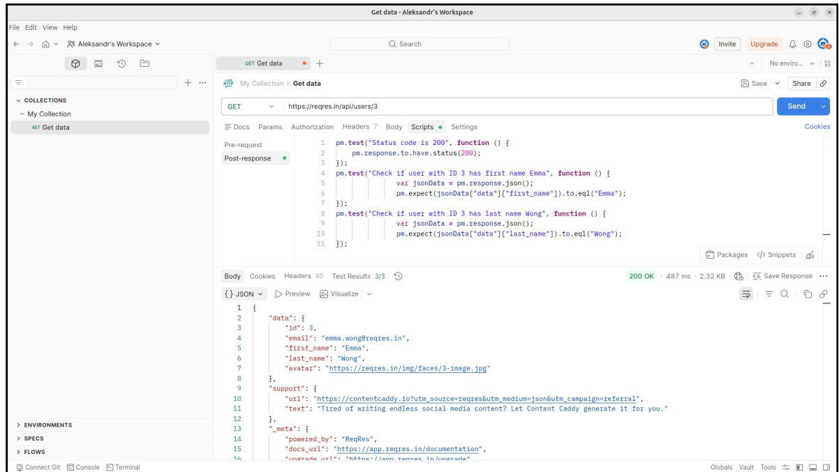
Рисунок 3 — Код тестов и ответ на GET-запрос
