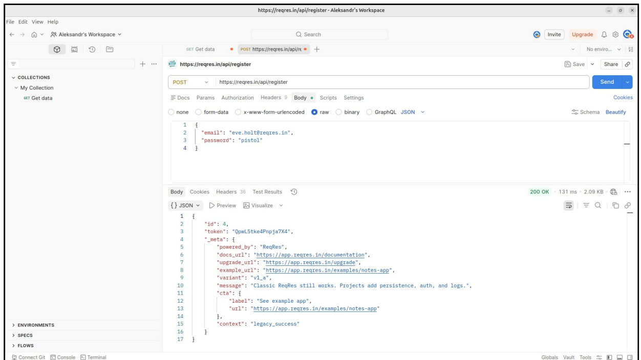
Рисунок 5 — POST-запрос и полученный ответ
