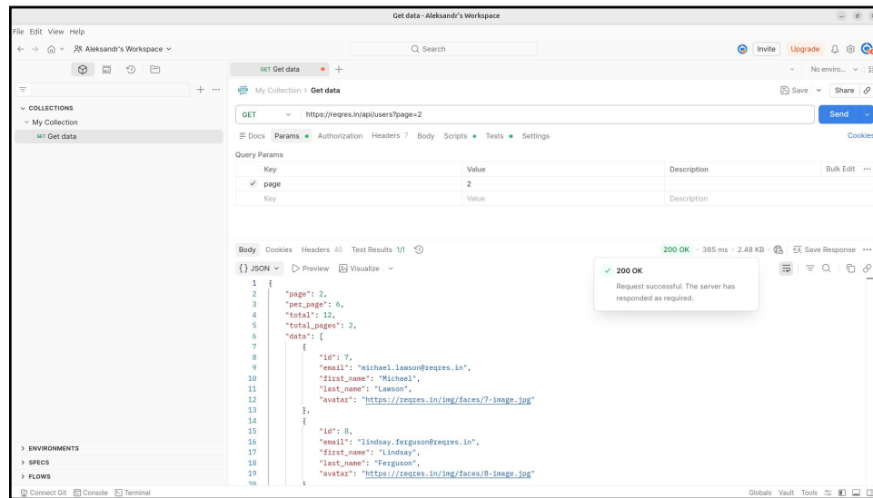
Рисунок 1 — GET-запрос и соответствующий ему ответ
