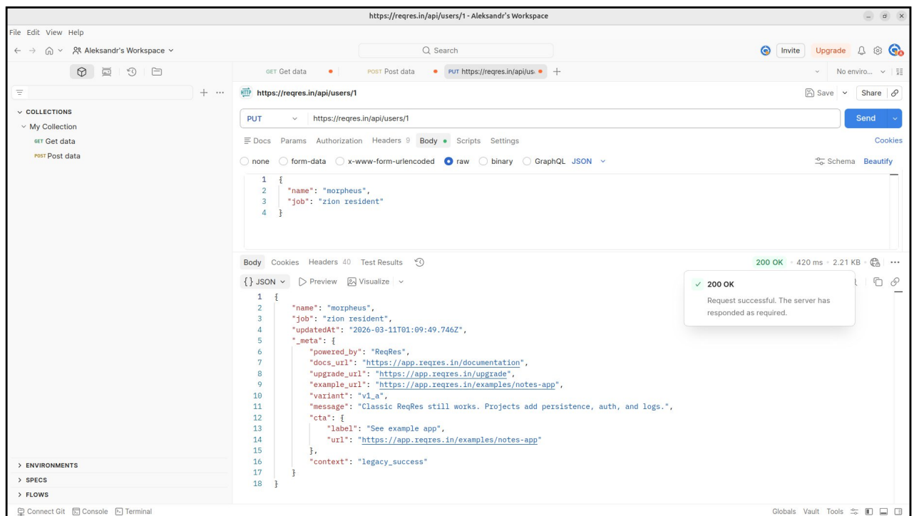
Рисунок 7 — PUT-запрос и полученный ответ
