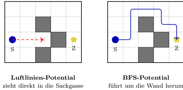
Abbildung 8: Minimalbeispiel einer dreiseitig umschlossenen Sackgasse (grau) zwischen Start S und Ziel Z. Links: Ein Potential auf Luftlinien-Distanz nimmt an jeder Position den kürzesten geometrischen Abstand zum Ziel und zieht den Agenten geradewegs in die Sackgasse, wo er endet (X), ohne die Wand einzurechnen. Rechts: Das in dieser Arbeit verwendete Potential auf BFS-Pfaddistanz kennt nur begehbare Wege und führt korrekt um die Wand herum. Schematische Darstellung, kein realer Weltausschnitt.
