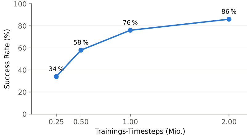
Abbildung 10: Lernkurve des historischen Referenzlaufs (ppo_lstm_curriculum, Bedingung C, Umgebung vor der v11-Revision; Curriculum-Phase 3, stochastische Evaluation auf 50 Seeds).
