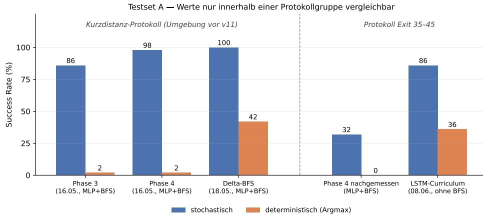
Abbildung 14: Entwicklung über die Modellgenerationen auf Testset A. Links die MLP-Baselines mit BFS-Orakel in der Observation, rechts der LSTM-Agent ohne Orakel. Die beiden Gruppen sind nicht miteinander vergleichbar: Die Mai-Messungen entstanden auf der Umgebung vor der v11-Revision unter einem Kurzdistanz-Protokoll, die Juni-Messungen unter dem Standardprotokoll (Exit 35–45). Wie groß der Unterschied ist, zeigt der vierte Balken: Dasselbe Phase-4-Modell fällt unter dem Standardprotokoll von 98 % auf 32 % stochastisch und von 2 % auf 0 % deterministisch. Nur die beiden rechten Balken tragen den Vergleich in Tabelle 9. Erzeugt mit scripts/plot_entwicklung.py .
