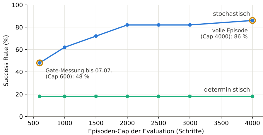
Abbildung 17: Erfolgsquote desselben Modells (bester Phase-1-Checkpoint, Seed 0) in Abhängigkeit des Episodenlimits der Evaluation, 50 Val-Seeds. Erzeugt mit scripts/plot_etappe6_figures.py .
