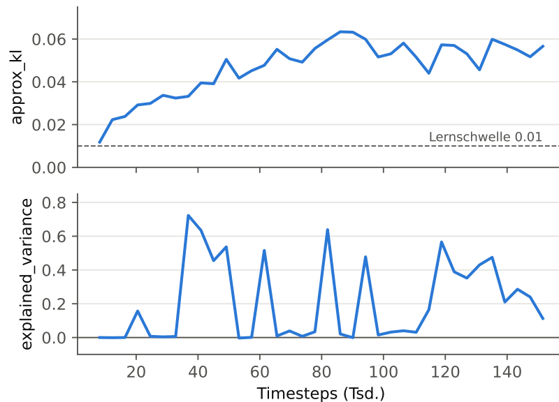
Abbildung 21: Validierungslauf batch_size=64 (Phase-1-Setup, Env v11), Stand 06.07.: approx_kl und explained_variance über der Zeit. Zur späteren Widerlegung dieses Befunds siehe Abschnitt 9.6.
