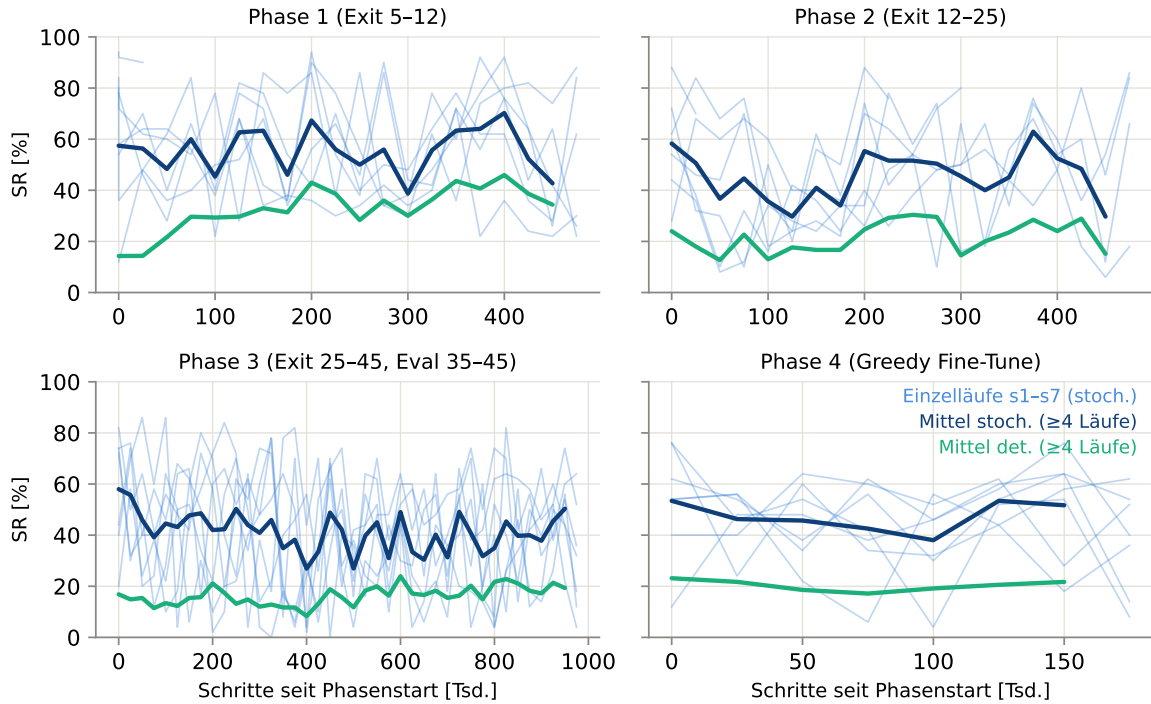
Abbildung 12: Trainingsverläufe der sieben v12-Läufe auf den Validierungs-Seeds 6000–6049, getrennt nach Curriculum-Phase. Dünne Linien: stochastische Erfolgsquote der Einzelläufe; dicke Linien: Ensemble-Mittel stochastisch (dunkelblau) und deterministisch (grün). Da die Schwierigkeit je Phase verschieden ist, sind die Werte nur innerhalb eines Panels vergleichbar. Die x-Achse zählt die Evaluationspunkte im 25k-Raster ab null; das letzte Panel endet deshalb bei 175k, obwohl das Phasenbudget 200k beträgt und ausgeschöpft wurde (Tabelle 11).
