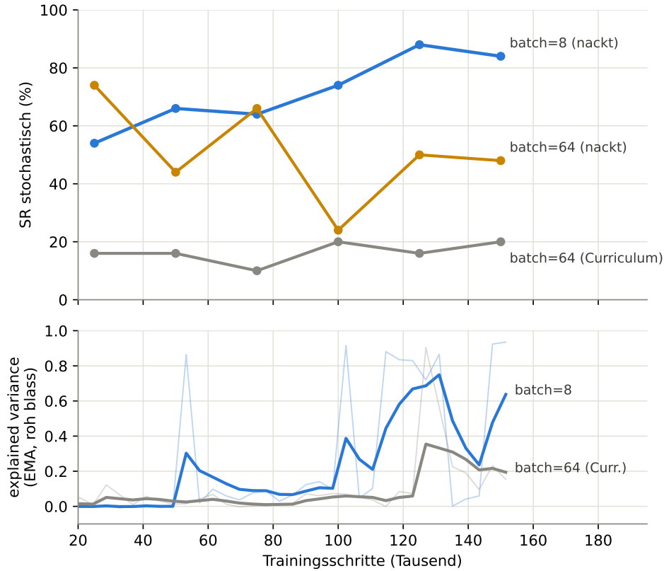
Abbildung 18: Batch-Größen-Forensik (alle Läufe Seed 1, Phase-1-Setup, 50 Val-Seeds, Limit 4000). Oben: stochastische Erfolgsquote. Unten: explained_variance des Critics, EMA-geglättet mit blassen Rohkurven. Erzeugt mit scripts/plot_etappe6_figures.py .
