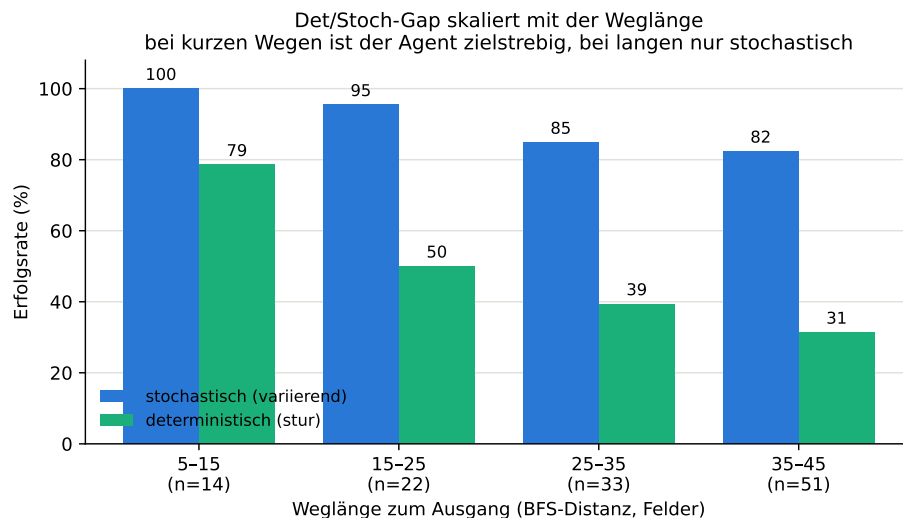
Abbildung 13: Erfolgsquote nach Startdistanz zum Exit (120 Welten des Validierungsbereichs, Seeds 6000–6119, finales v12-Modell, Limit 4000): Die deterministische SR fällt kontinuierlich mit der Weglänge, die stochastische bleibt hoch. Erzeugt mit scripts/plot_det_gap_distanz.py .
