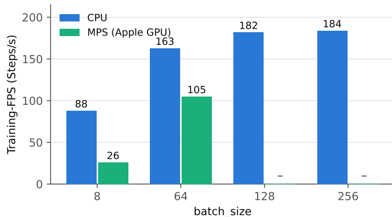
Abbildung 20: Training-FPS nach Device und Batch-Größe (RecurrentPPO, 16 Umgebungen, Apple M-Serie). MPS wurde für \text{batch} \geq 128 nicht weiter gemessen, da bereits bei 64 unterlegen.
