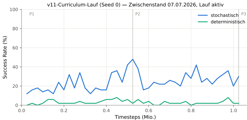
Abbildung 11: Lernkurve des ersten v11-Gesamtlaufs (Seed 0, Zwischenstand in Phase 3), beide Betriebsarten. Vertikale Linien: Phasenwechsel; die x-Achse ist über die Phasen kumuliert. Erzeugt mit scripts/plot_run_curve.py .
