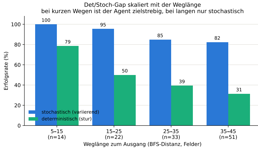
Abbildung 9: Erfolgsquote nach Startdistanz zum Exit (120 Welten des Validierungsbereichs, Seeds 6000–6119, finales v12-Modell, Limit 4000): Die deterministische SR fällt kontinuierlich mit der Weglänge, die stochastische bleibt hoch. Erzeugt mit scripts/plot_det_gap_distanz.py .
