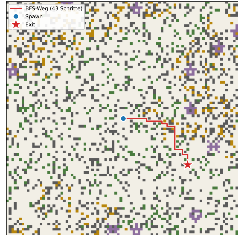
Fertige Welt mit kürzestem Weg (Stufe 3 + Exit-Platzierung)
