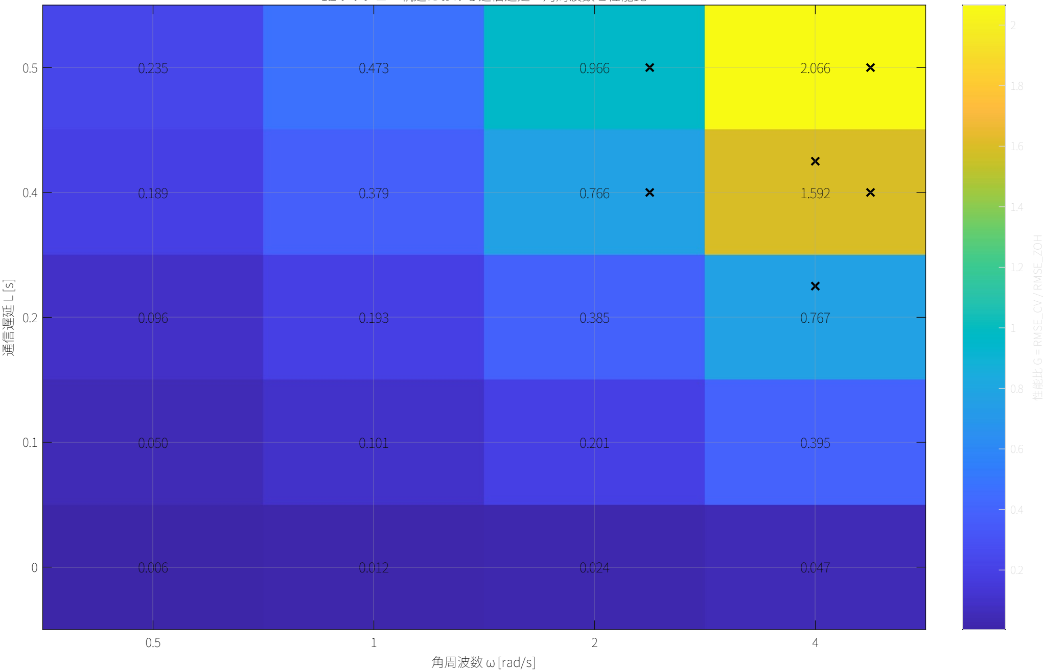
1:2リサージュ軌道における通信遅延・角周波数と性能比
