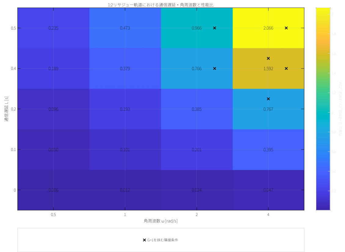
図 6 1:2 リサージュ軌道における通信遅延・角周波数と性能比
