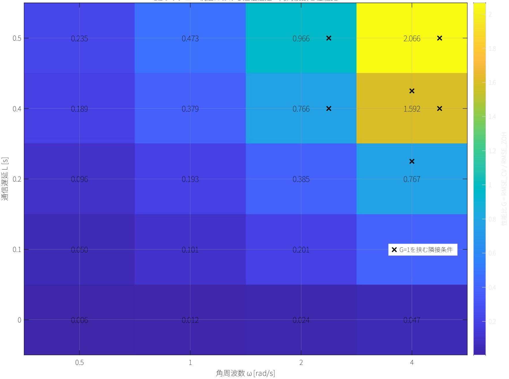
1:2リサージュ軌道における通信遅延・角周波数と性能比
