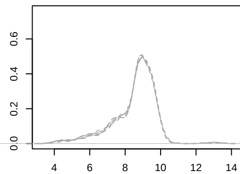
CycLoess
