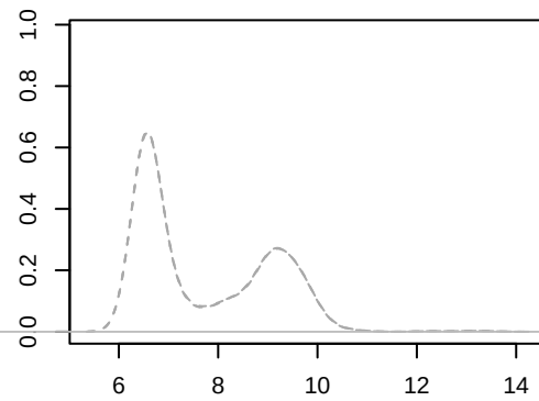
VSN
