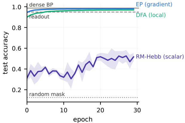
MNIST
