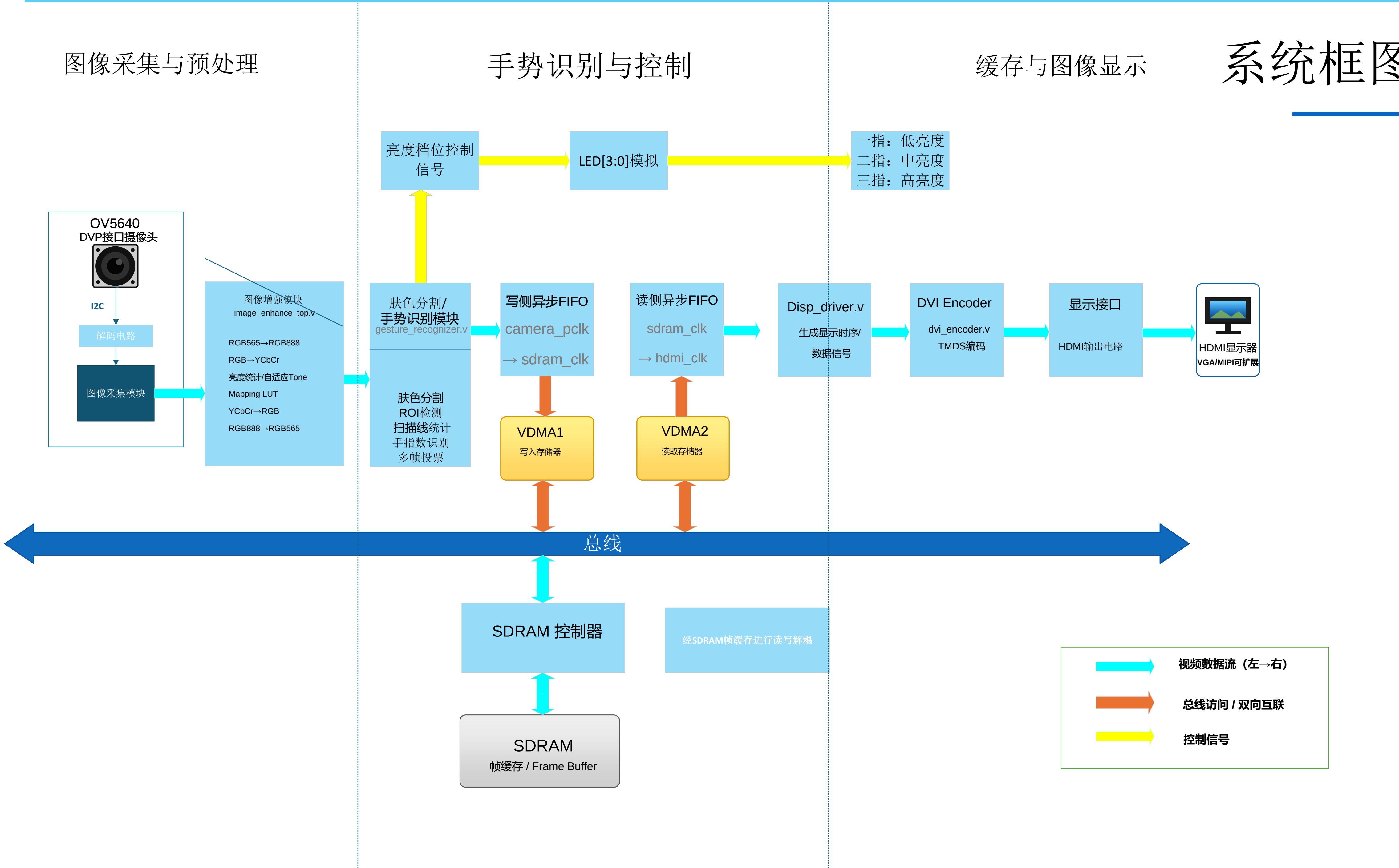
系统框图 —— 基于FPGA视觉手势识别的牙科诊疗灯亮度控制
