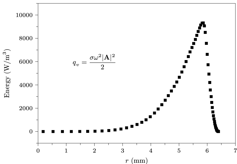
图 3.1 内热源沿径向的分布
