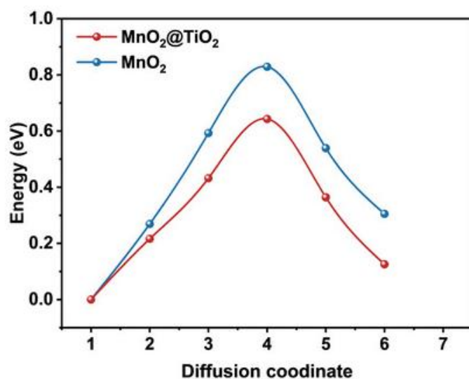
图 3-1 MnO@TiO 中 Zn 迁移及扩散势垒
