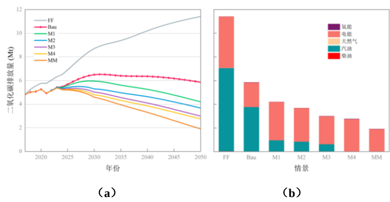
图 3-2 不同情景下上海市乘用车的温室气体排放量
