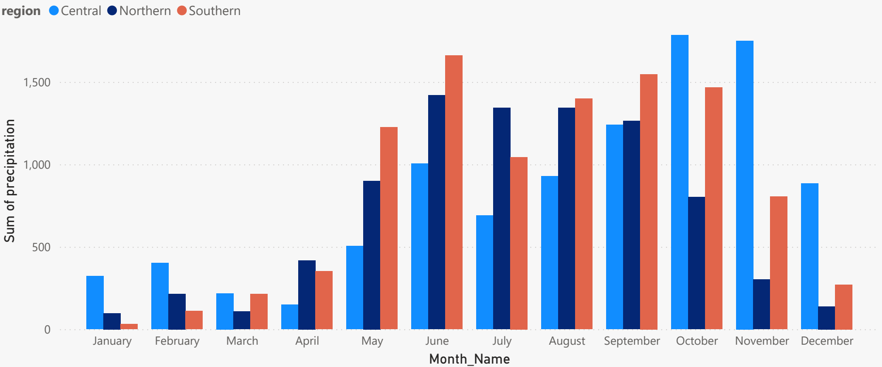
So sánh tổng lượng mưa theo tháng giữa 3 miền
