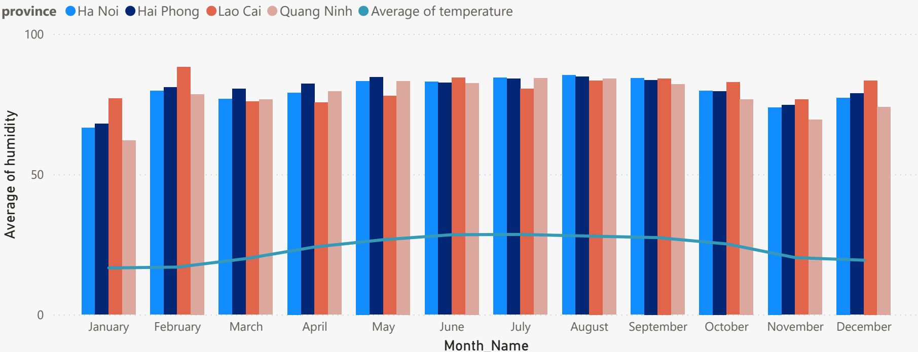
Mối tương quan giữa Nhiệt độ và Độ ẩm
