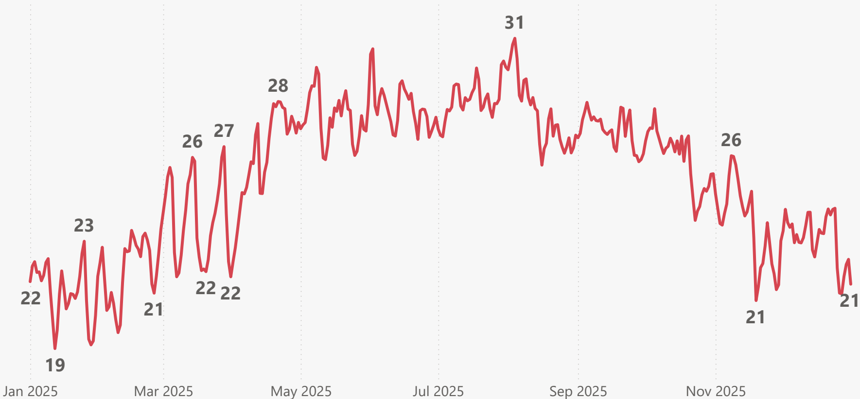
Biến động nhiệt độ trung bình theo thời gian
