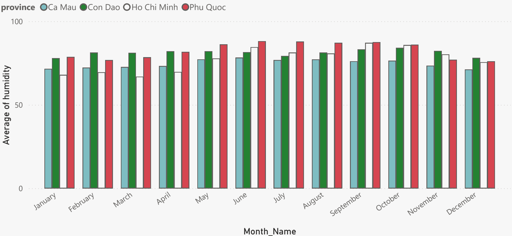
Độ ẩm trung bình theo tháng
