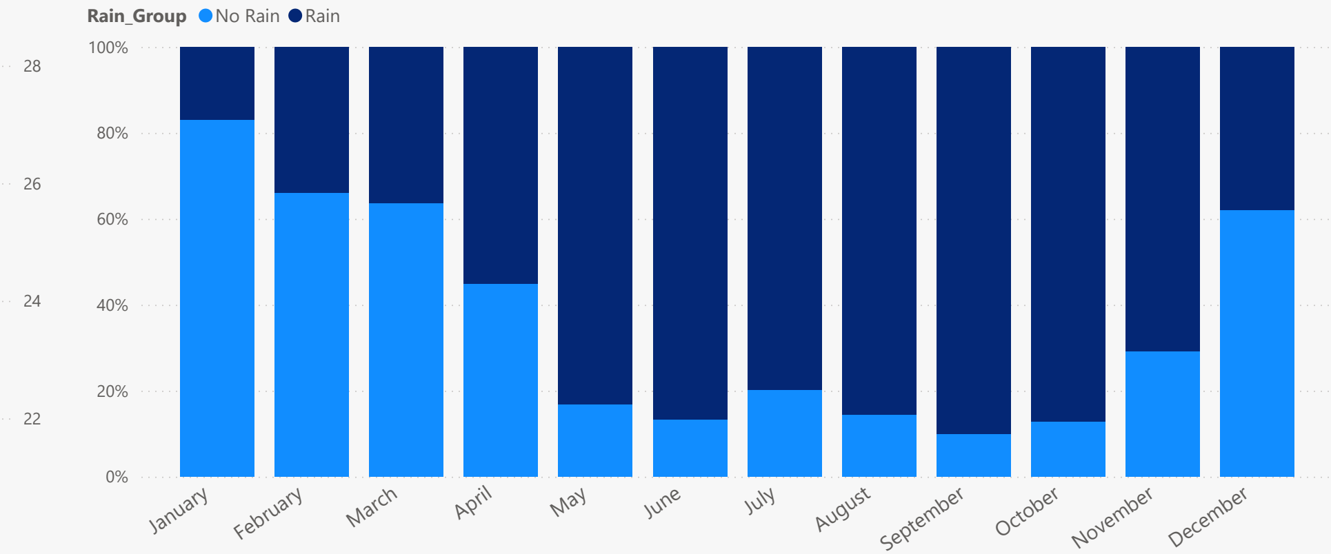
Tỷ lệ ngày Mưa vs ngày Không Mưa theo tháng
