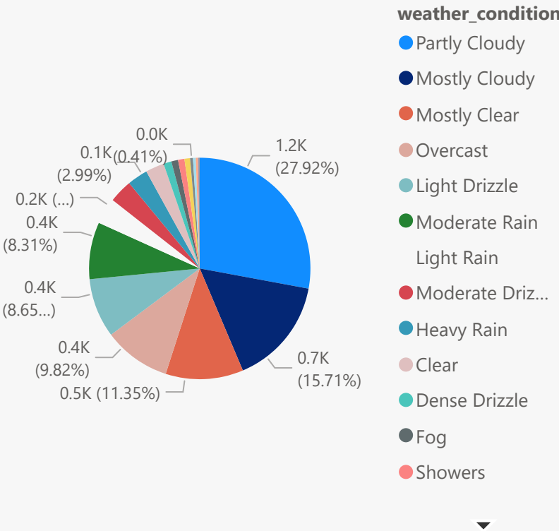
Tỷ lệ loại hình thời tiết
