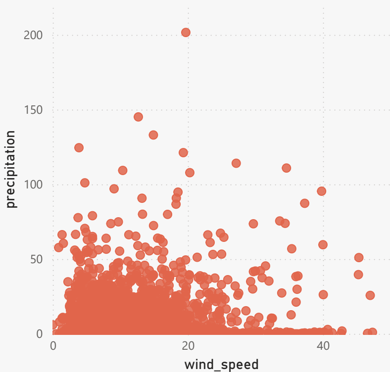
Tốc độ gió so với lượng mưa
