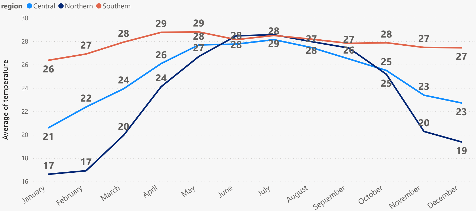
So sánh nhiệt độ trung bình hàng tháng giữa 3 miền
