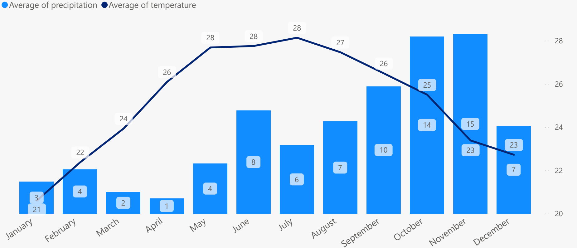
Trung bình nhiệt độ và lượng mưa
