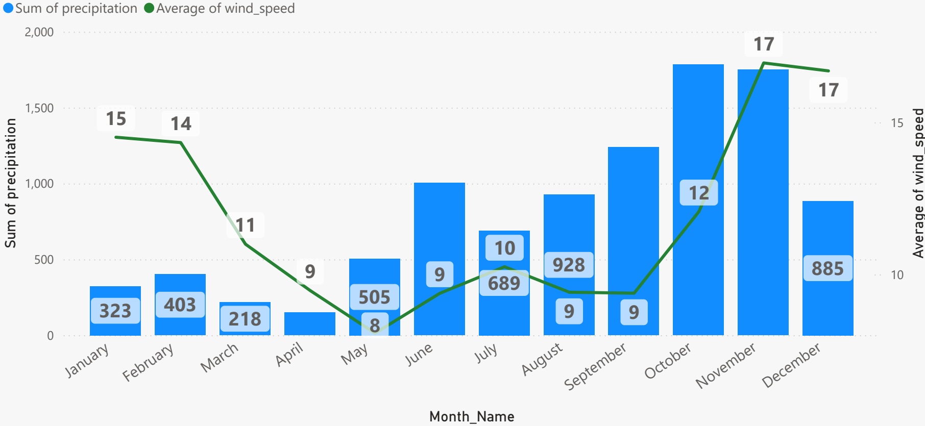
Mối liên hệ giữa Lượng mưa và Tốc độ gió
