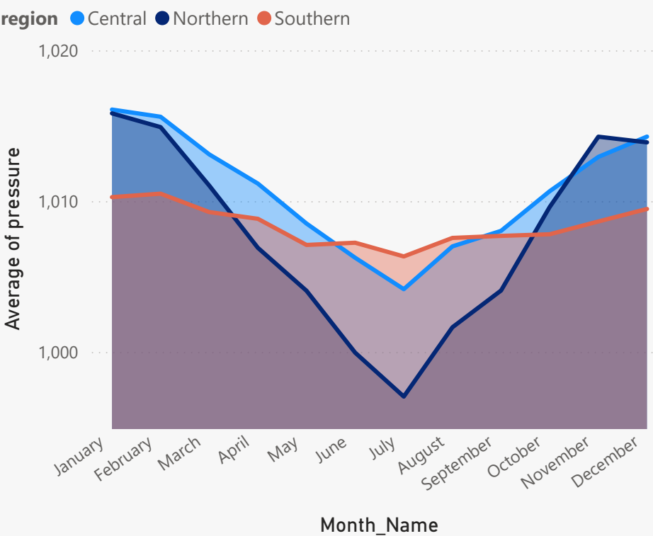
Biến thiên áp suất các miền theo từng tháng trong năm
