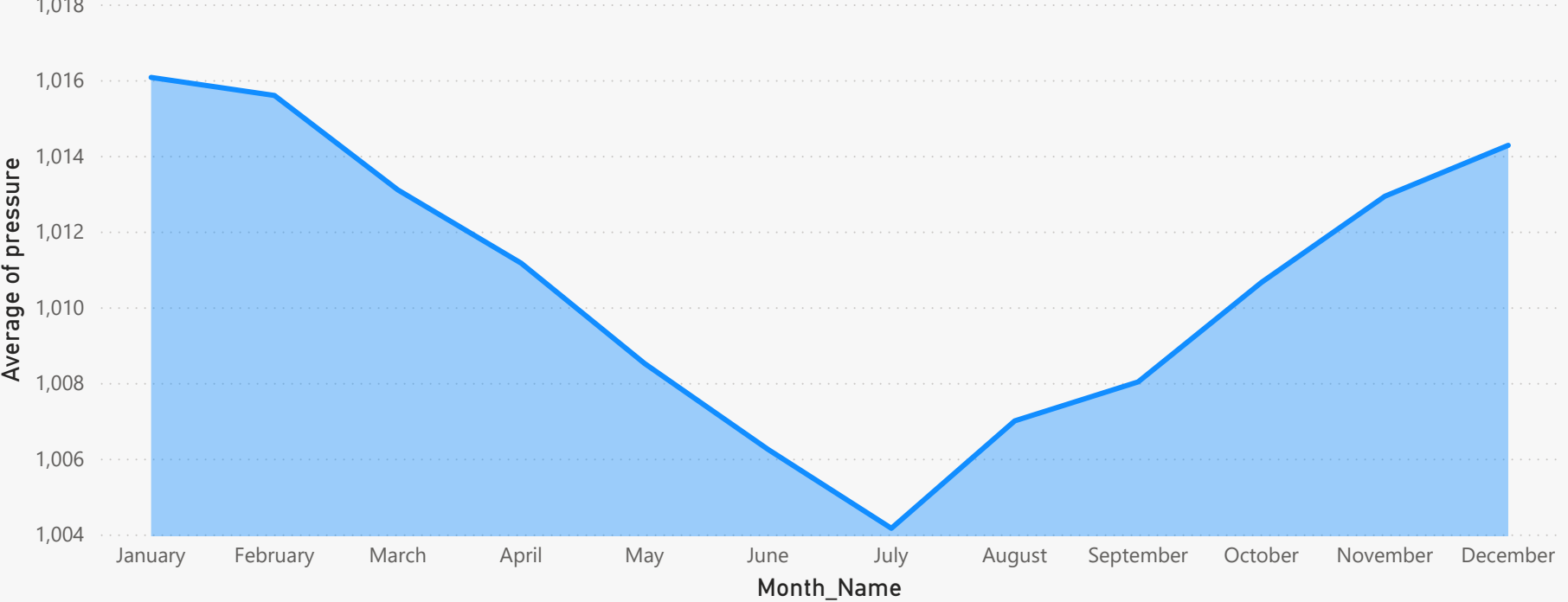
Diễn biến áp suất không khí (Pressure) trong năm
