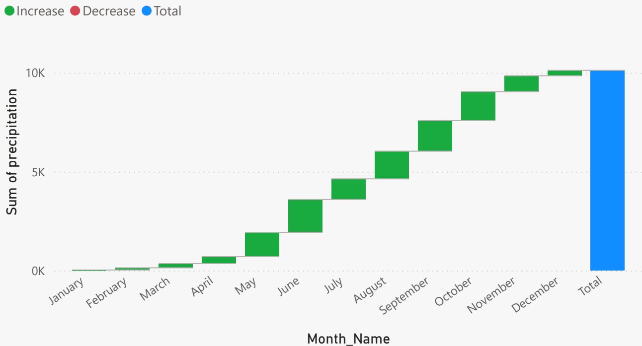
Tích lũy lượng mưa từ đầu năm đến cuối năm
