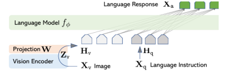
(d) LLaVA projector-based design [7].
