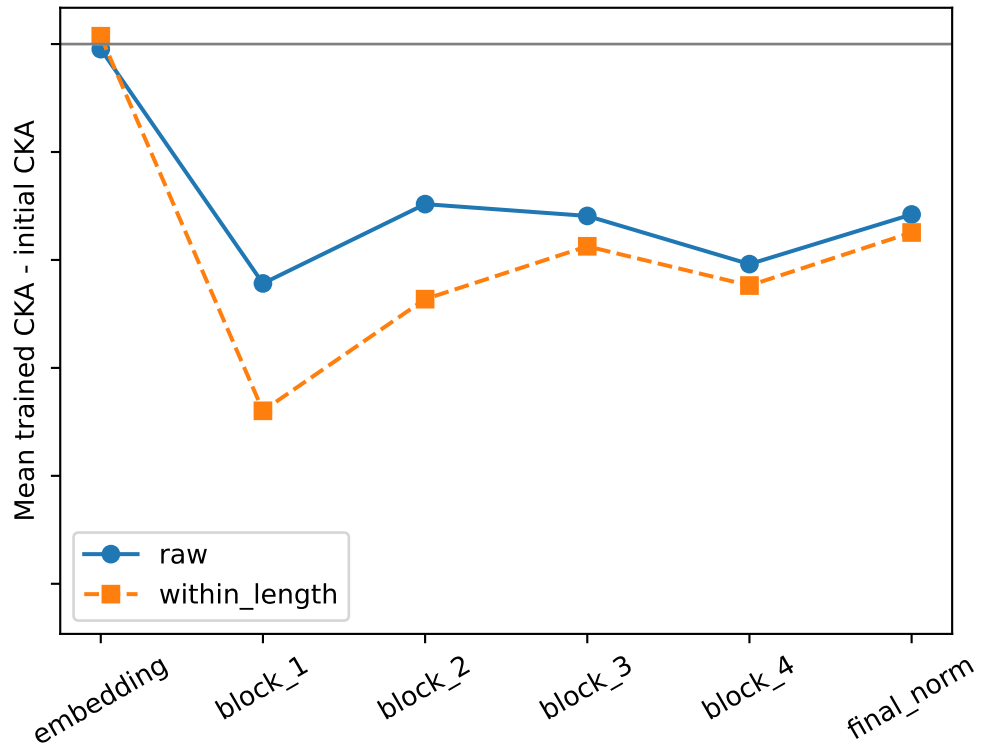
prefix_mean
