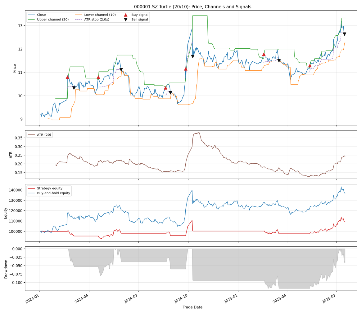
图5 平安银行海龟策略回测图（20/10通道）
