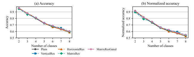
图 3: 从二分类到八分类的合成缩放, 对五个图族与四种算子取平均。
