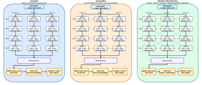
图 1: 分支–层网络上各残差邻域的架构概览。消息传递骨干与图层级读出保持不变，仅改变残差路径。
