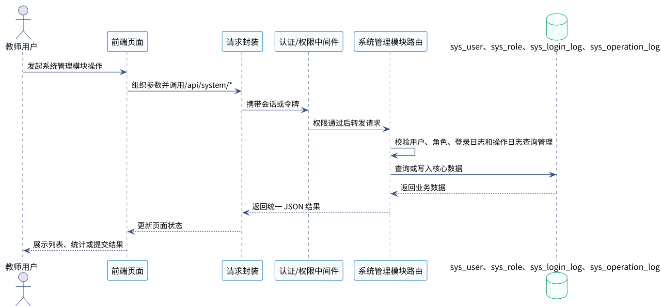
图 5-36 系统管理模块时序 UML 图
