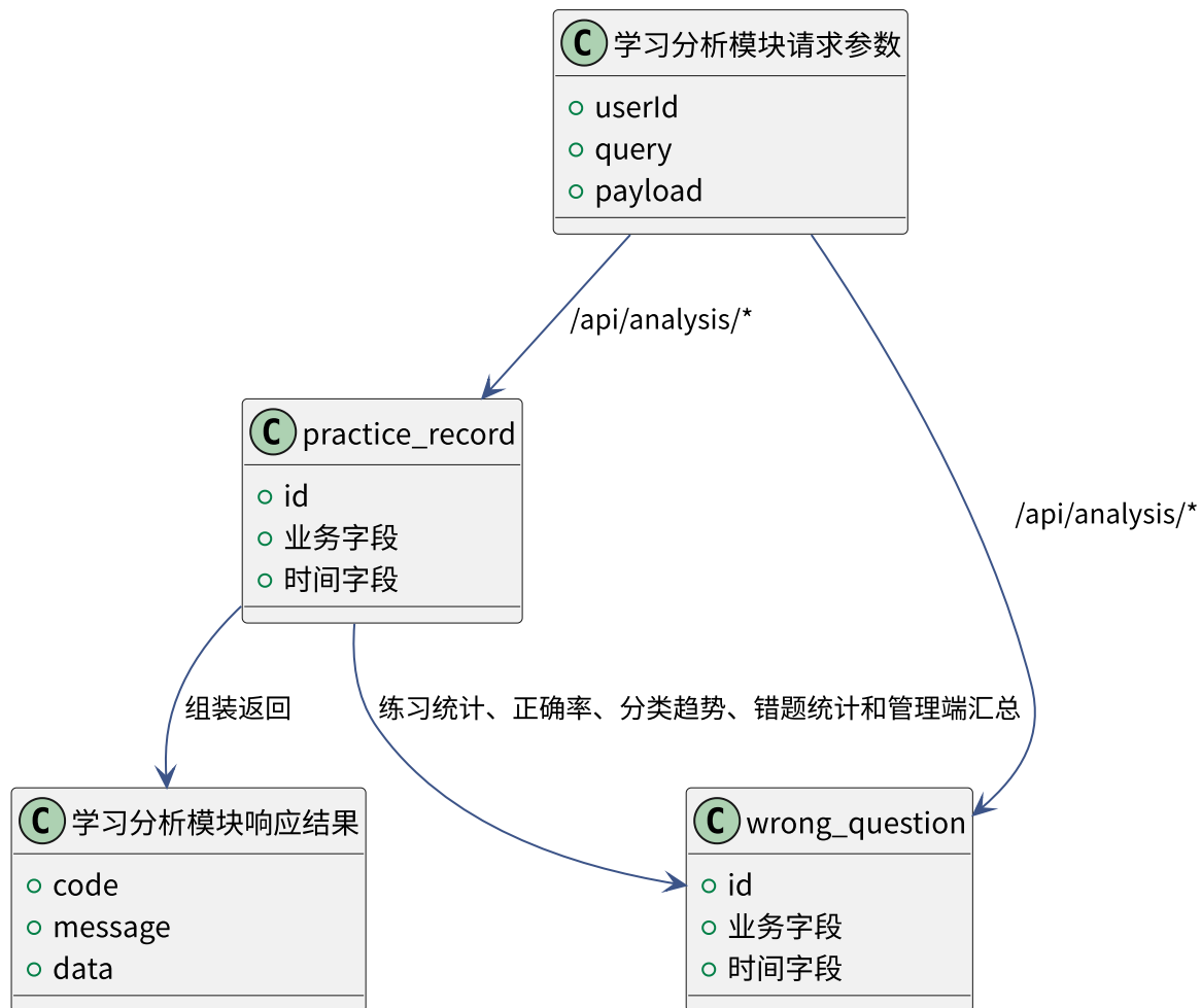
图 5-34 学习分析模块数据关系 UML 图
