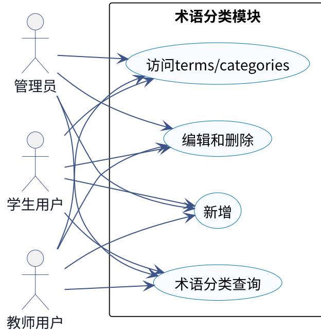
图 5-11 术语分类模块用例 UML 图
