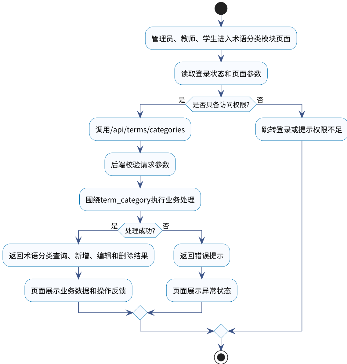
面向越南留学生的铁道专业汉越术语翻译学习软件术语分类模块活动图
