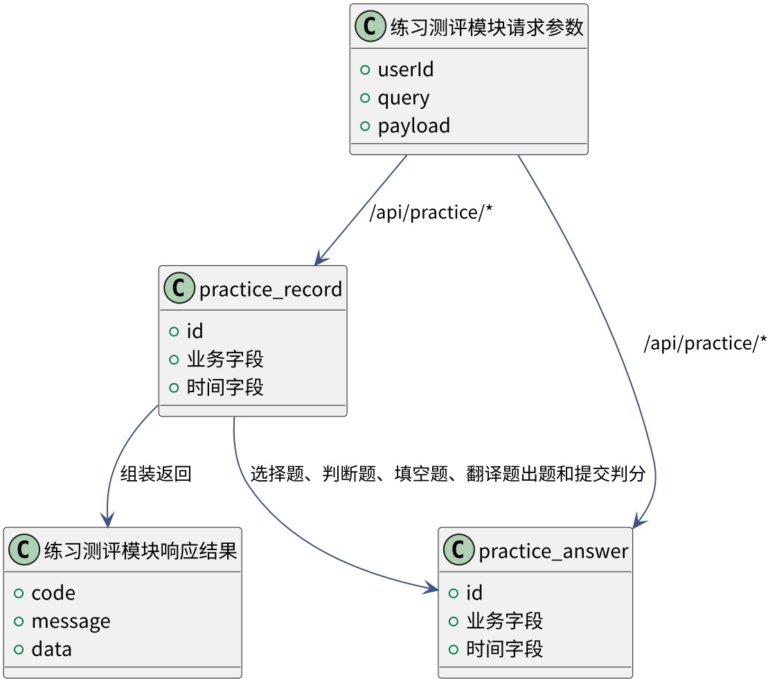
图 5-28 练习测评模块数据关系 UML 图
