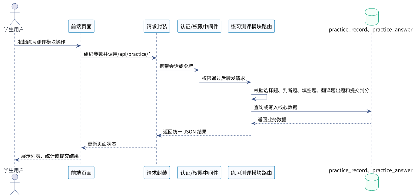
面向越南留学生的铁道专业汉越术语翻译学习软件练习测评模块时序图
