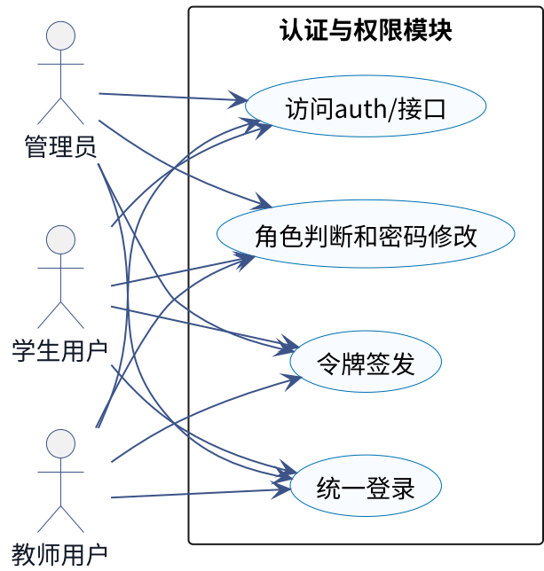
图 5-5 认证与权限模块用例 UML 图
