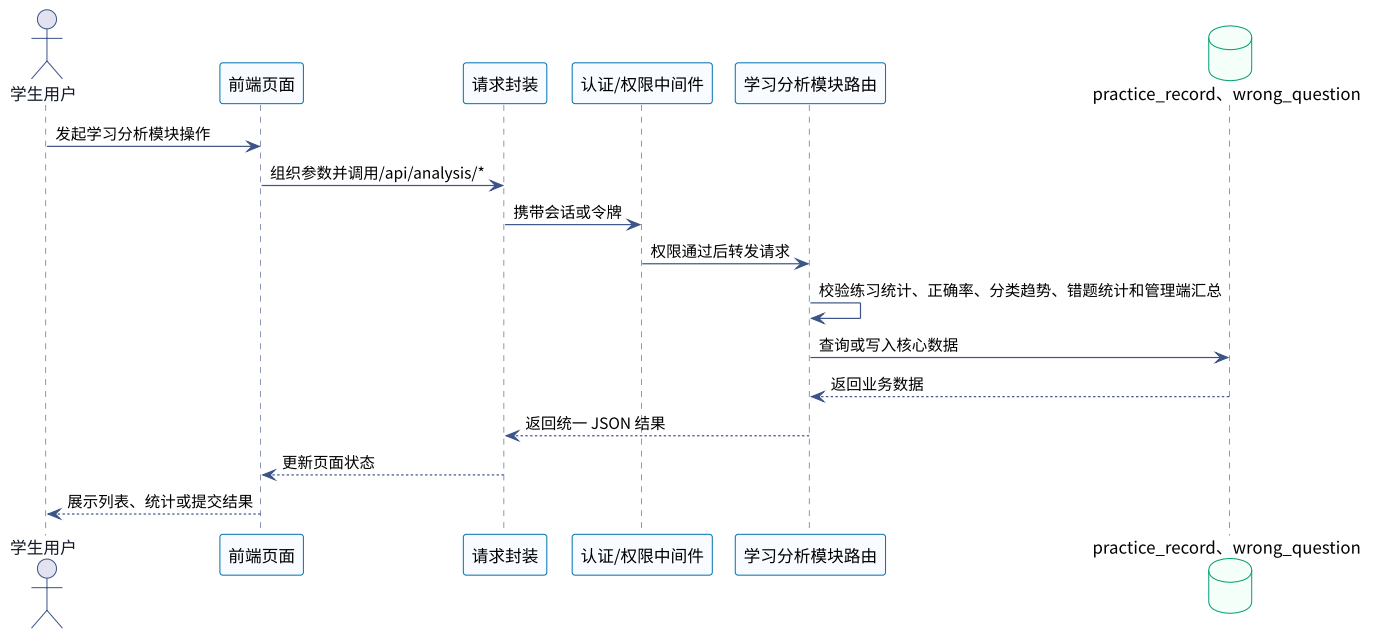
图 5-30 学习分析模块时序 UML 图
