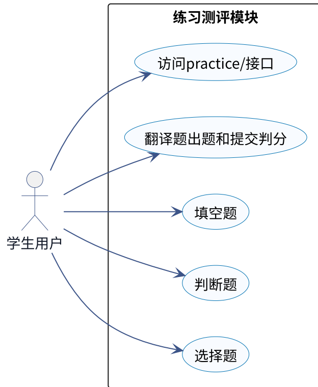
图 5-23 练习测评模块用例 UML 图
