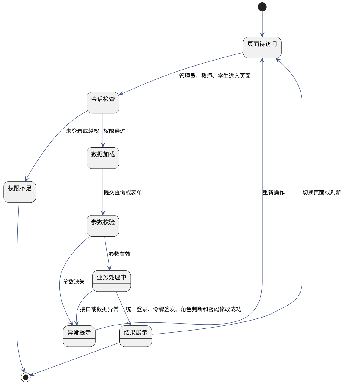
图 5-8 认证与权限模块状态 UML 图
