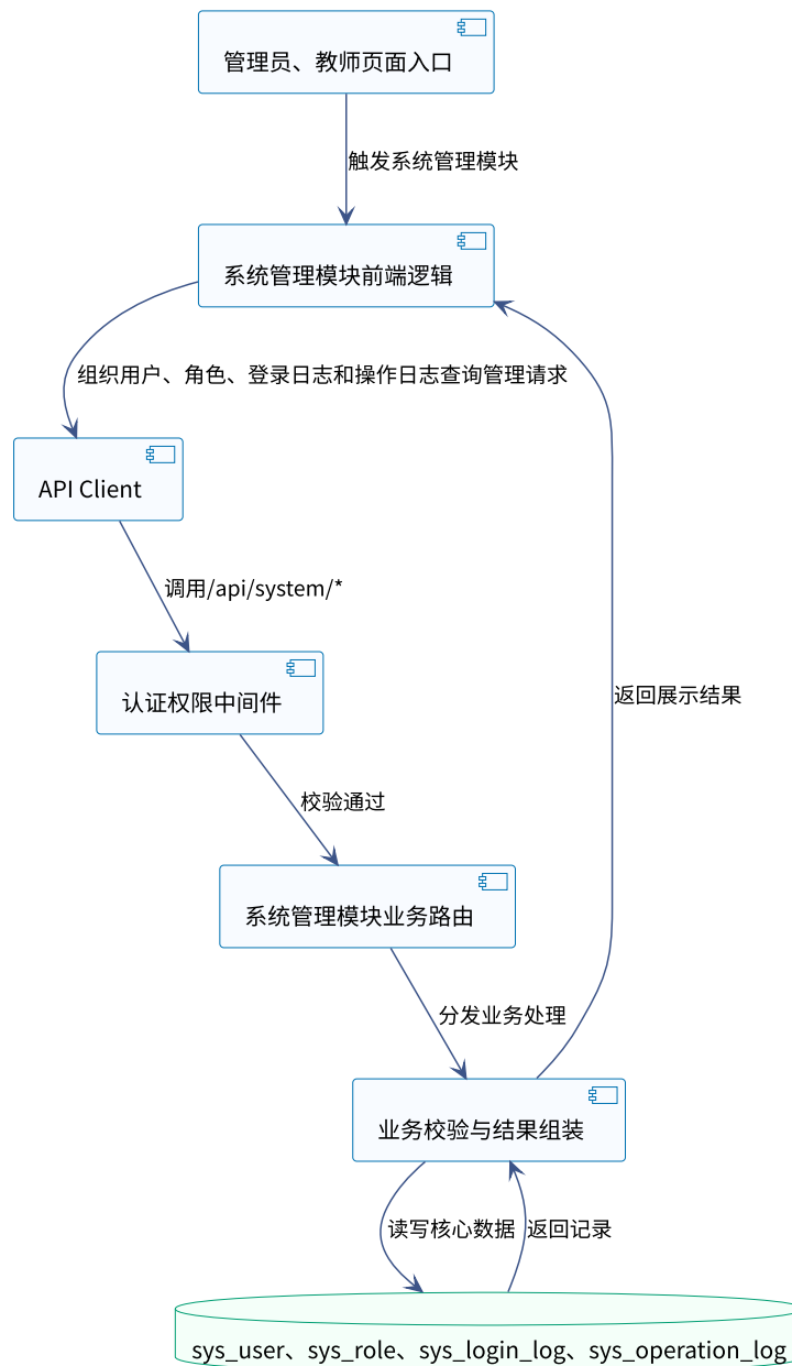
面向越南留学生的铁道专业汉越术语翻译学习软件系统管理模块组件协作图
