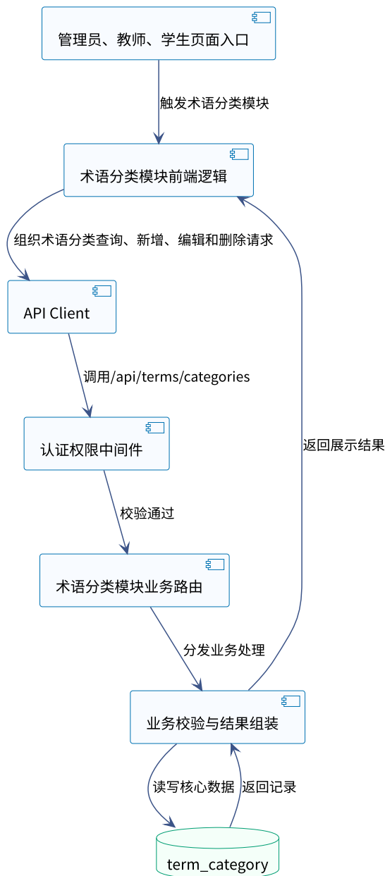
面向越南留学生的铁道专业汉越术语翻译学习软件术语分类模块组件协作图
