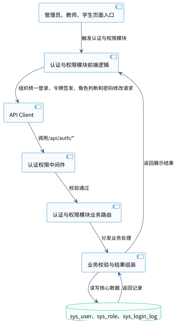
面向越南留学生的铁道专业汉越术语翻译学习软件认证与权限模块组件协作图
