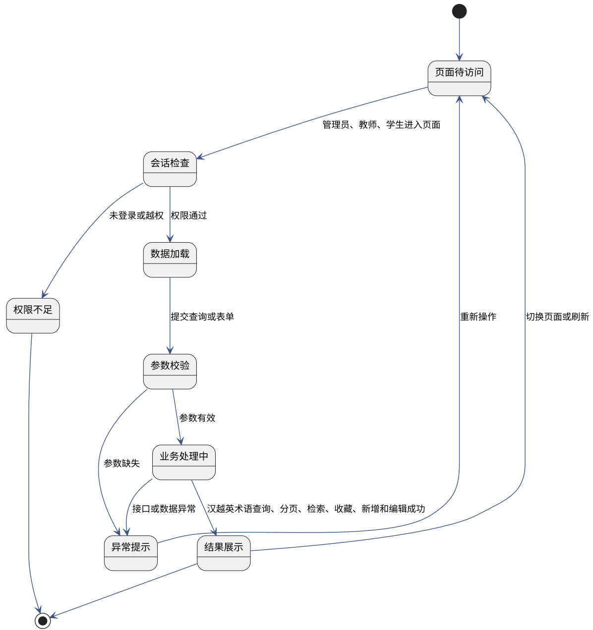
图 5-20 铁道术语模块状态 UML 图
