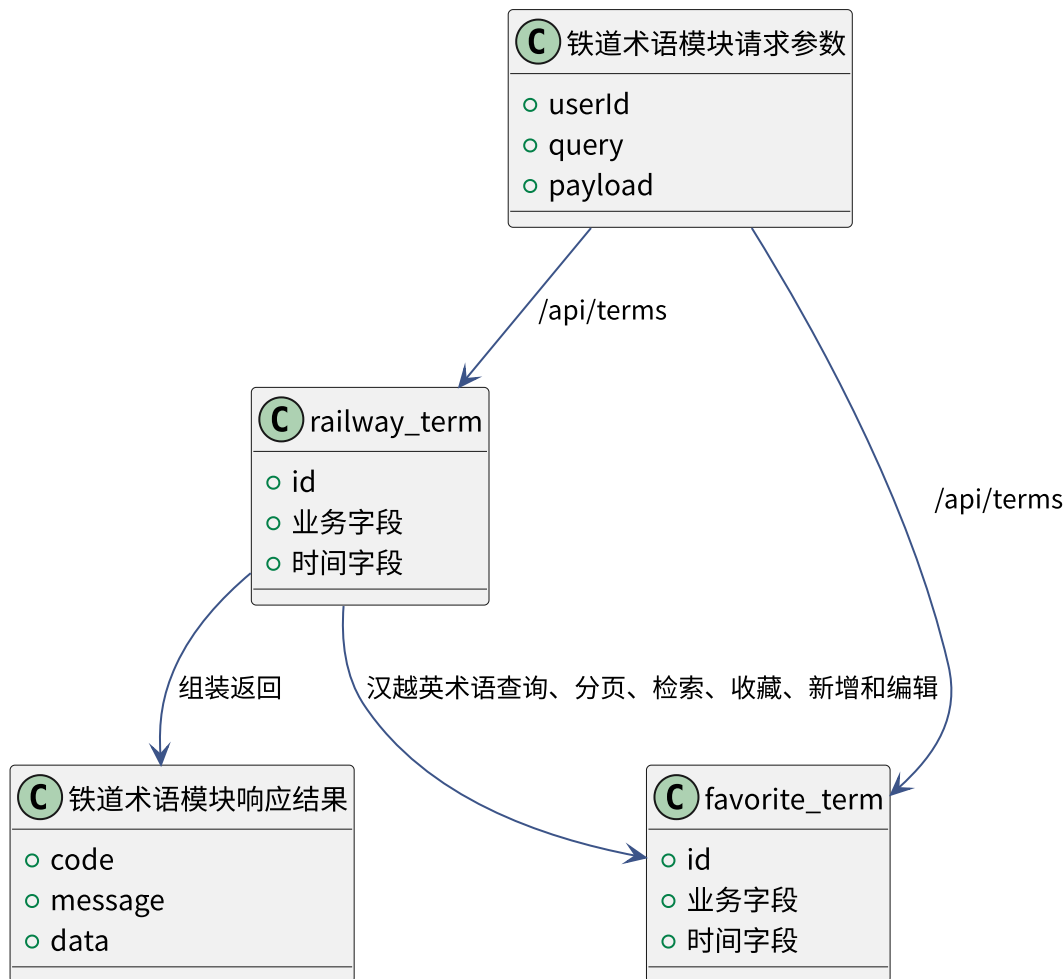
图 5-22 铁道术语模块数据关系 UML 图
