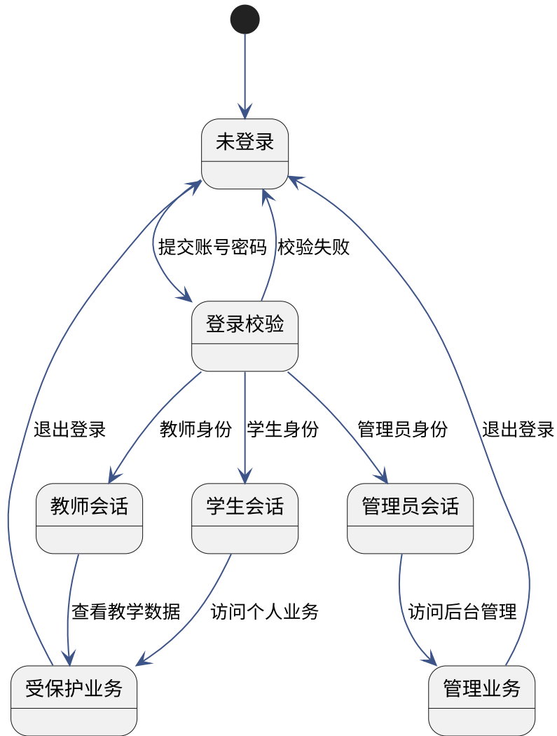
图 5-3 权限状态 UML 图
