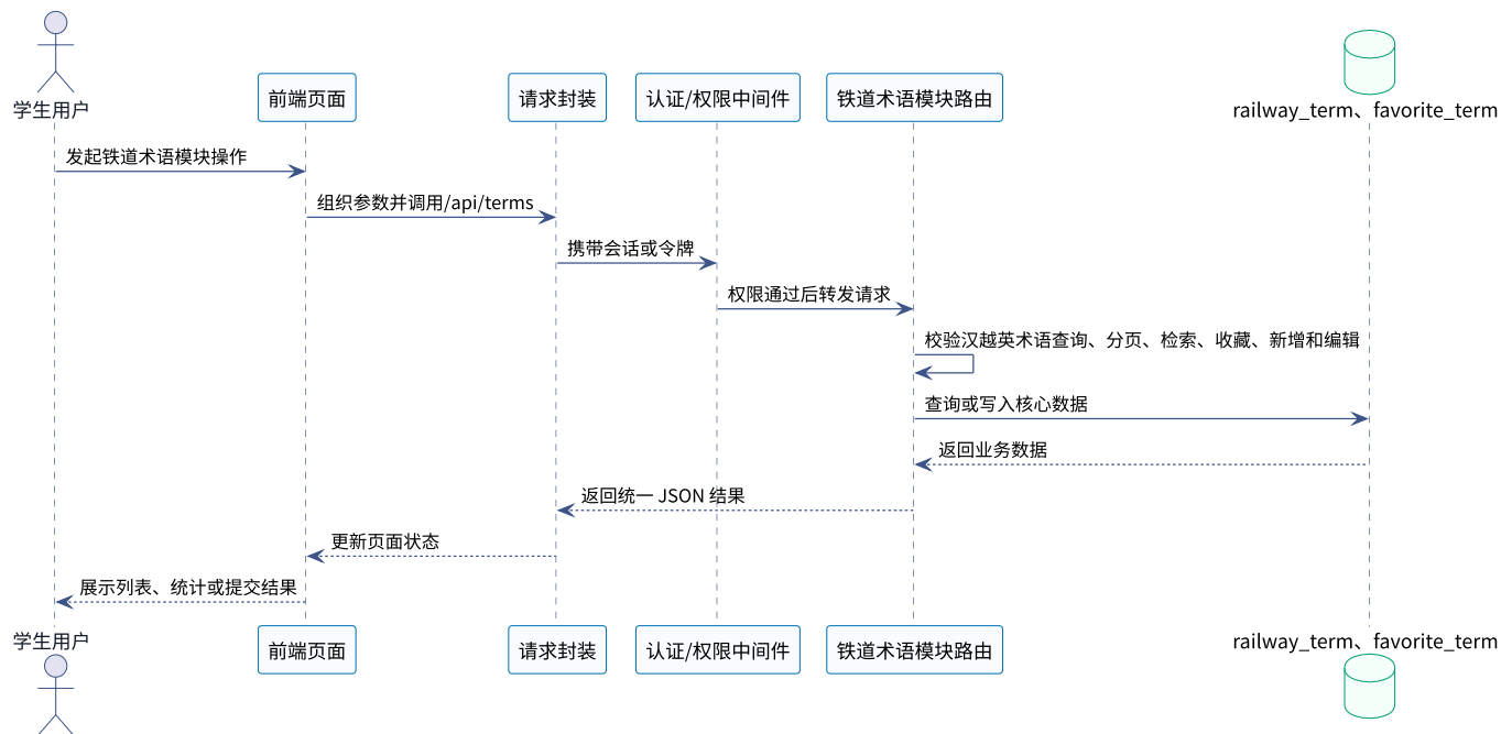
面向越南留学生的铁道专业汉越术语翻译学习软件铁道术语模块时序图
