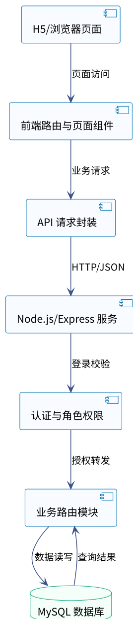
图 5-1 系统组件 UML 图
