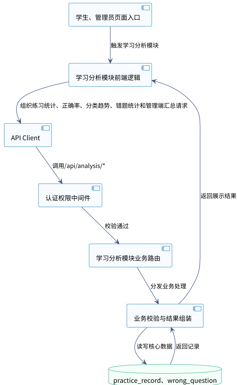
面向越南留学生的铁道专业汉越术语翻译学习软件学习分析模块组件协作图
