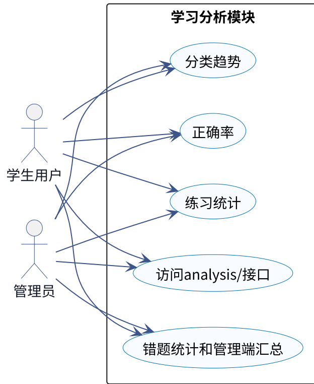
图 5-29 学习分析模块用例 UML 图
