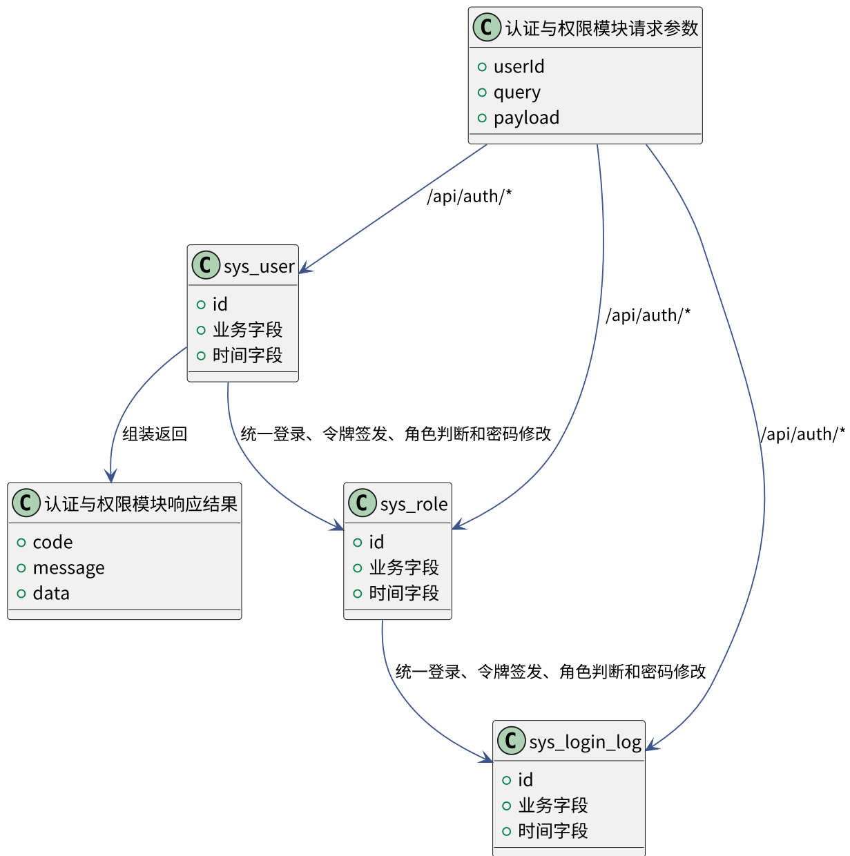
图 5-10 认证与权限模块数据关系 UML 图
