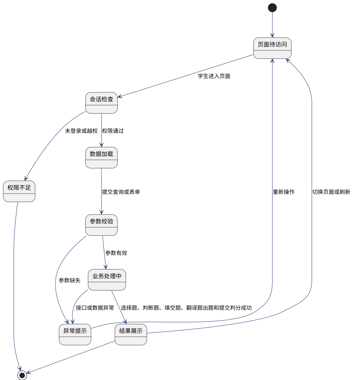
图 5-26 练习测评模块状态 UML 图
