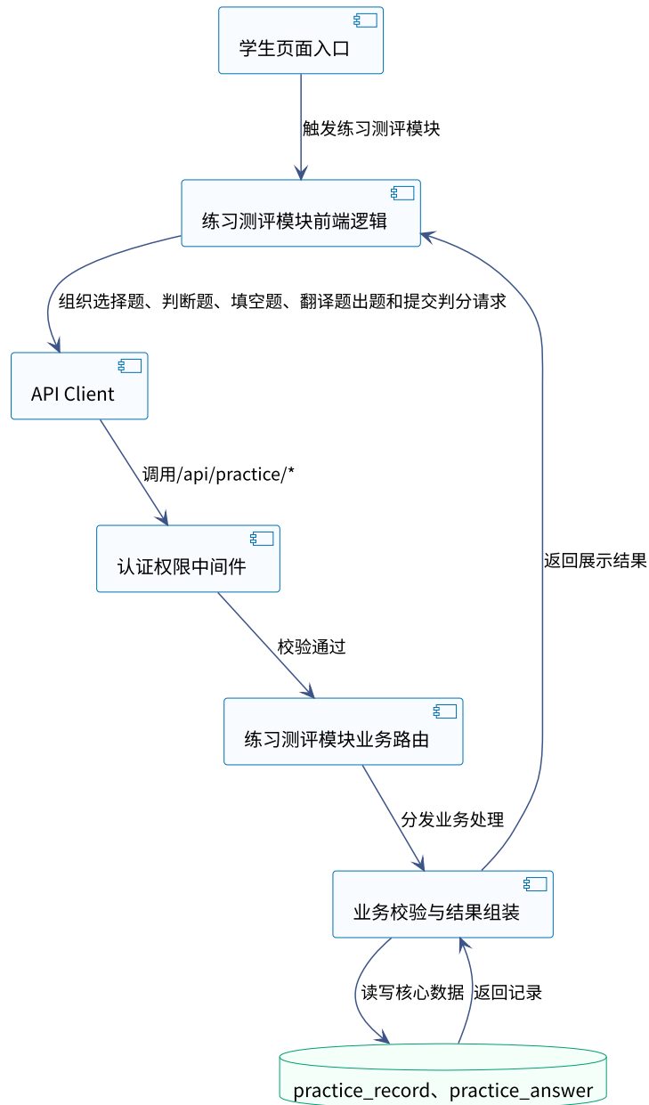
面向越南留学生的铁道专业汉越术语翻译学习软件练习测评模块组件协作图
