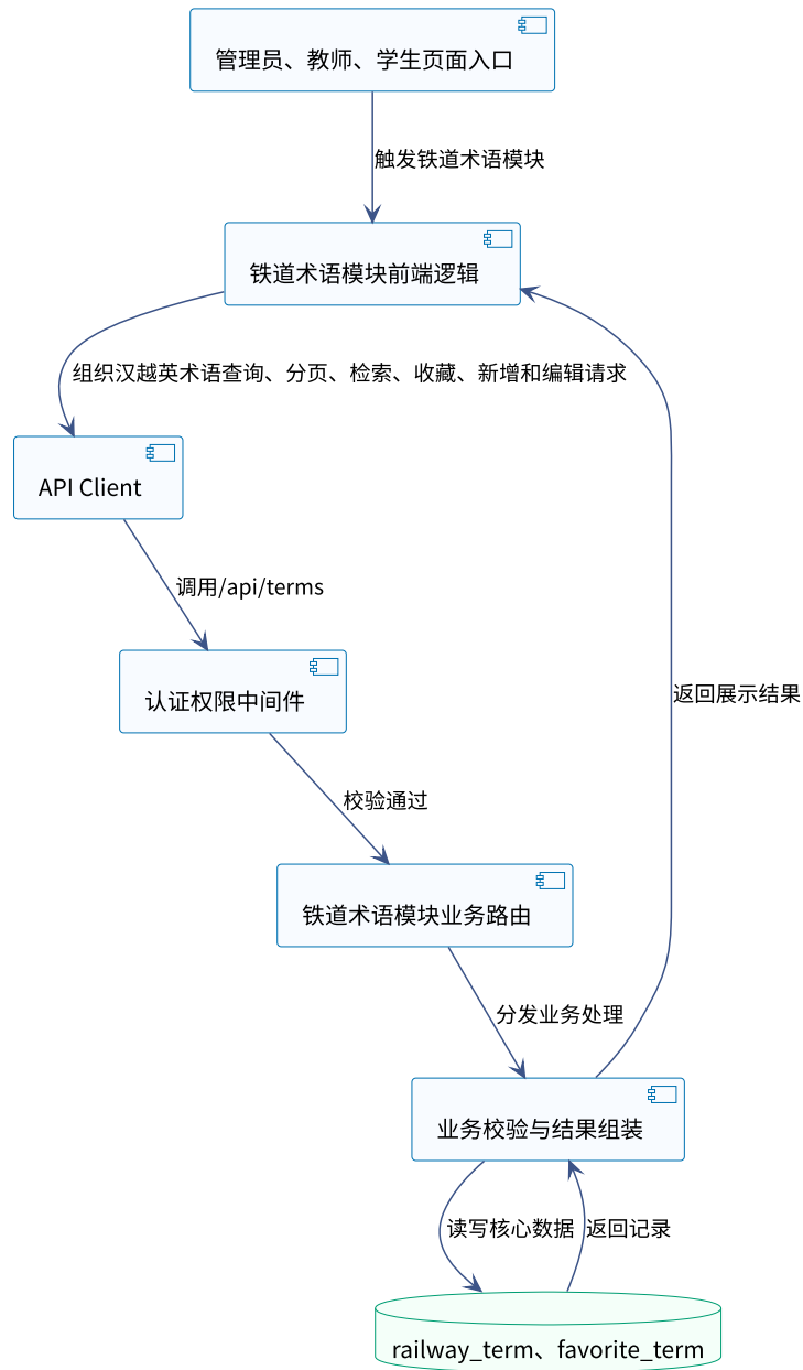
面向越南留学生的铁道专业汉越术语翻译学习软件铁道术语模块组件协作图
