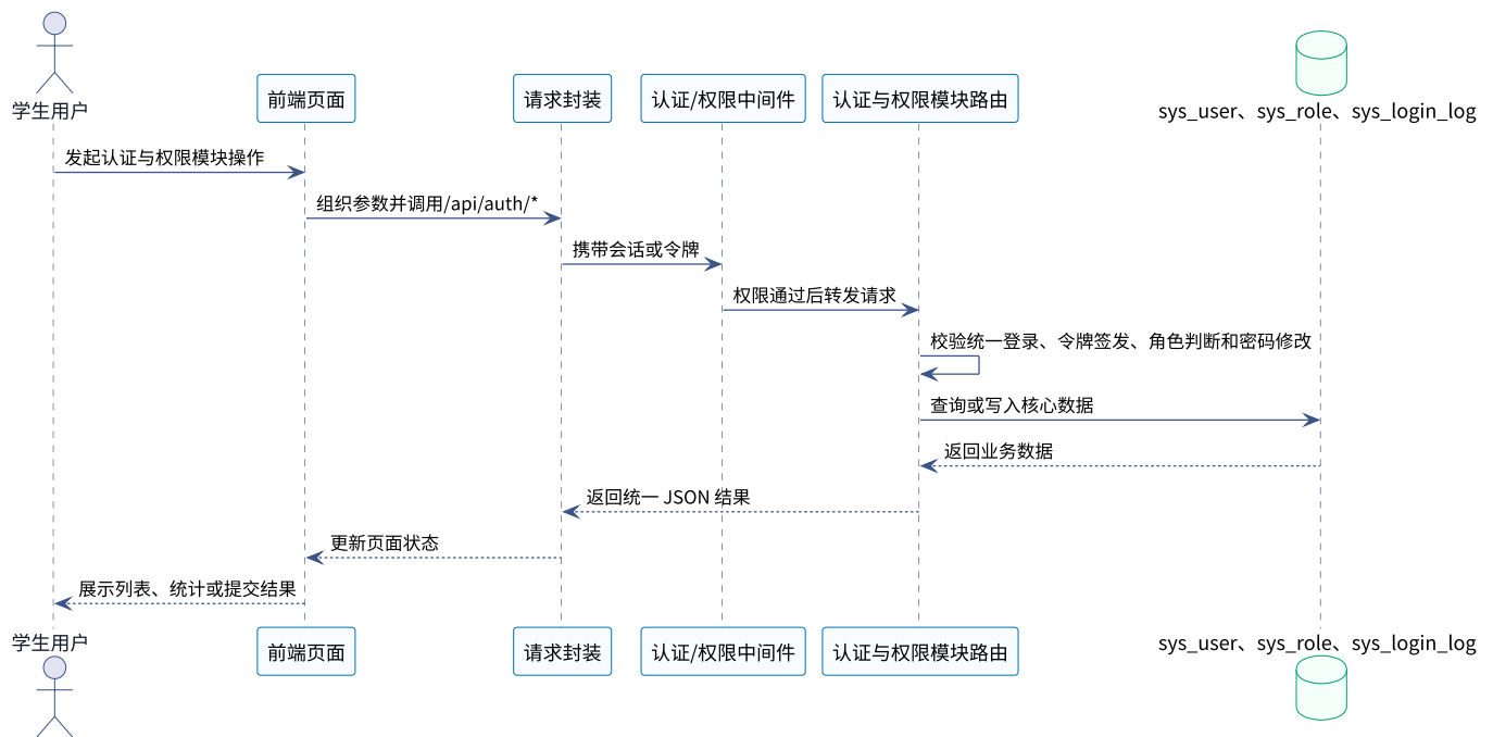
面向越南留学生的铁道专业汉越术语翻译学习软件认证与权限模块时序图
