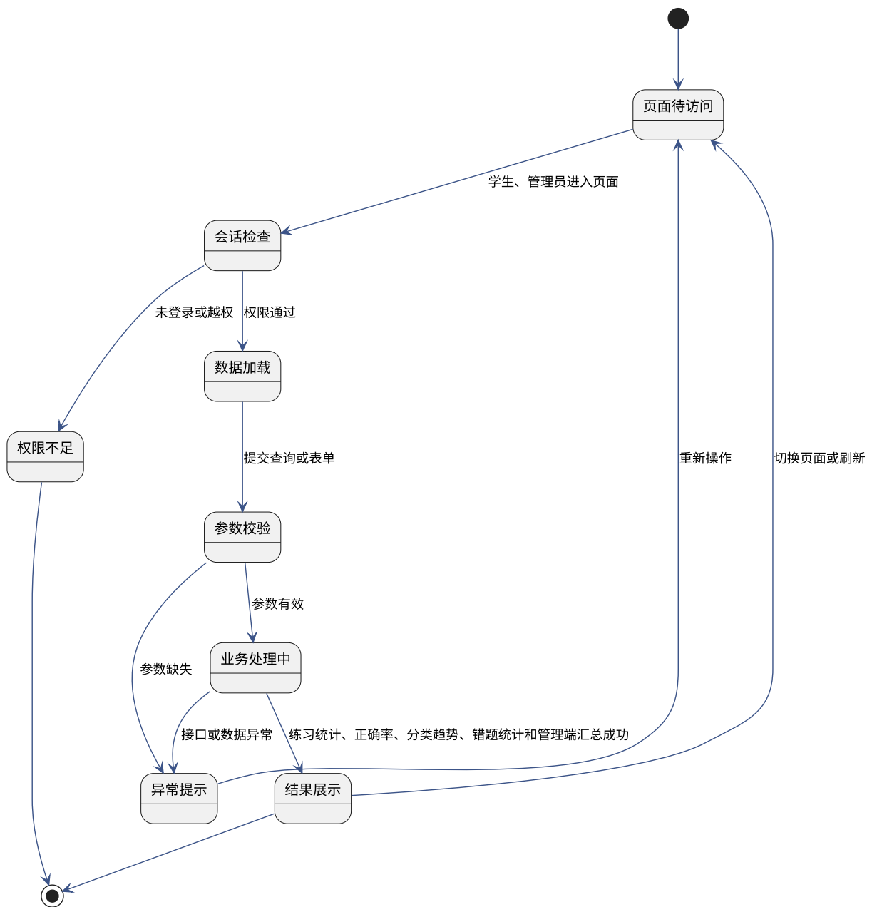
图 5-32 学习分析模块状态 UML 图
