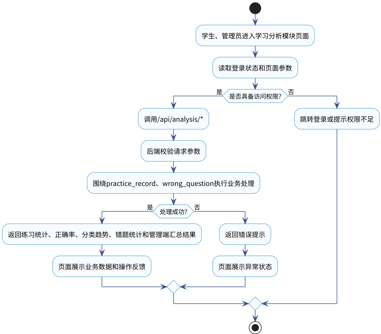
面向越南留学生的铁道专业汉越术语翻译学习软件学习分析模块活动图
