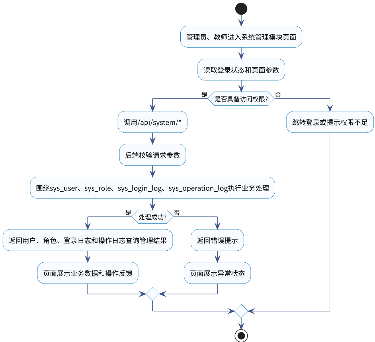
面向越南留学生的铁道专业汉越术语翻译学习软件系统管理模块活动图
