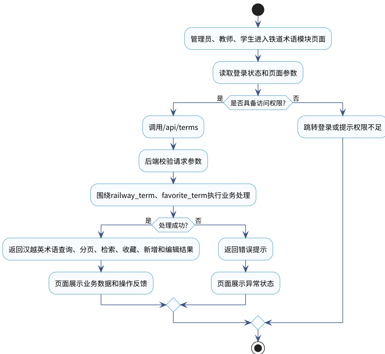
面向越南留学生的铁道专业汉越术语翻译学习软件铁道术语模块活动图
