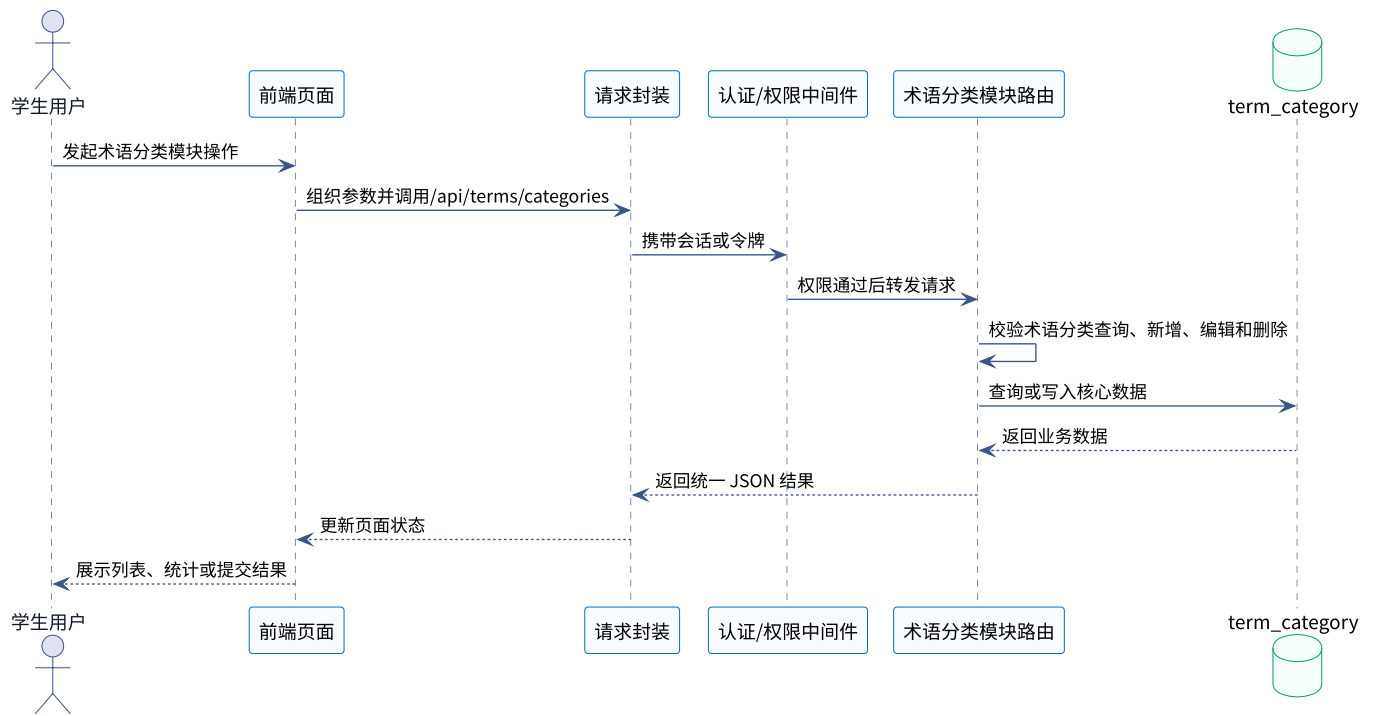
图 5-12 术语分类模块时序 UML 图
