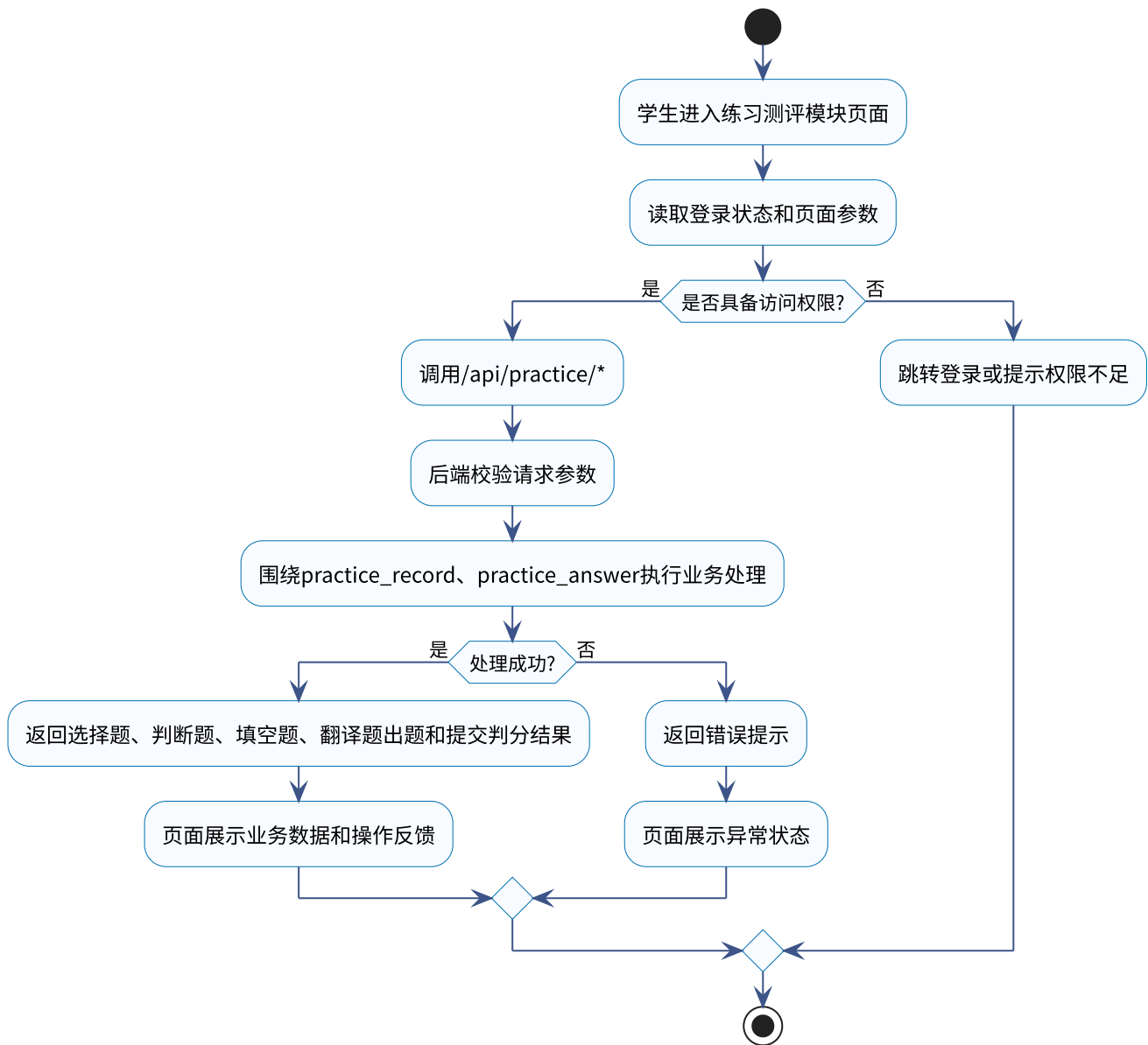
面向越南留学生的铁道专业汉越术语翻译学习软件练习测评模块活动图
