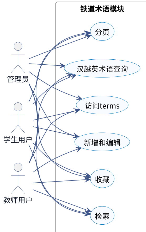
图 5-17 铁道术语模块用例 UML 图
