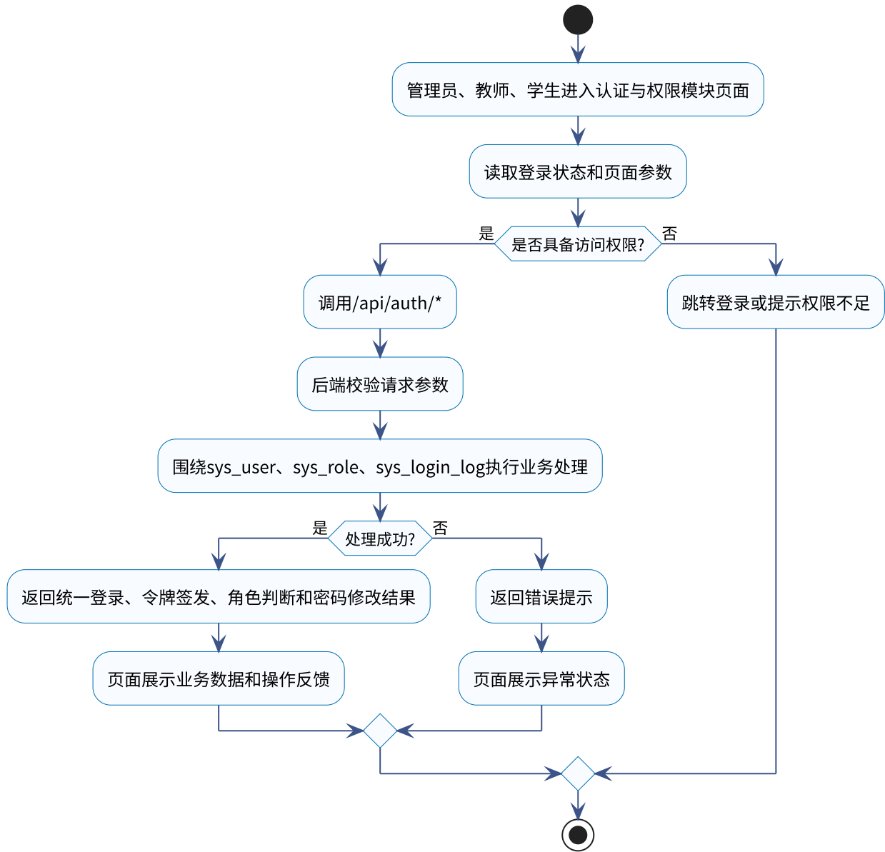
面向越南留学生的铁道专业汉越术语翻译学习软件认证与权限模块活动图
