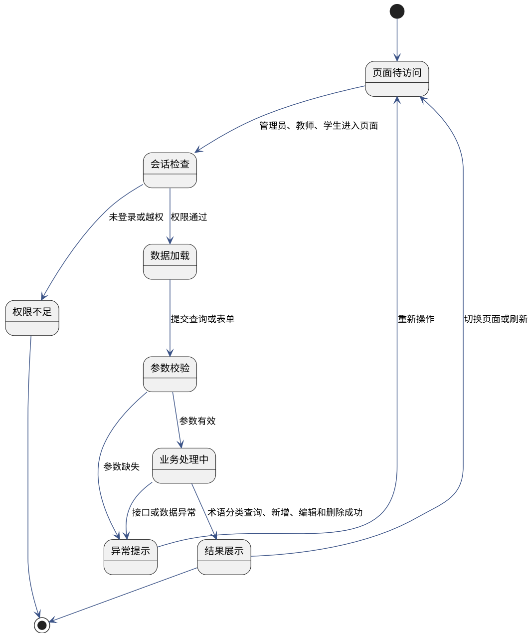
图 5-14 术语分类模块状态 UML 图
