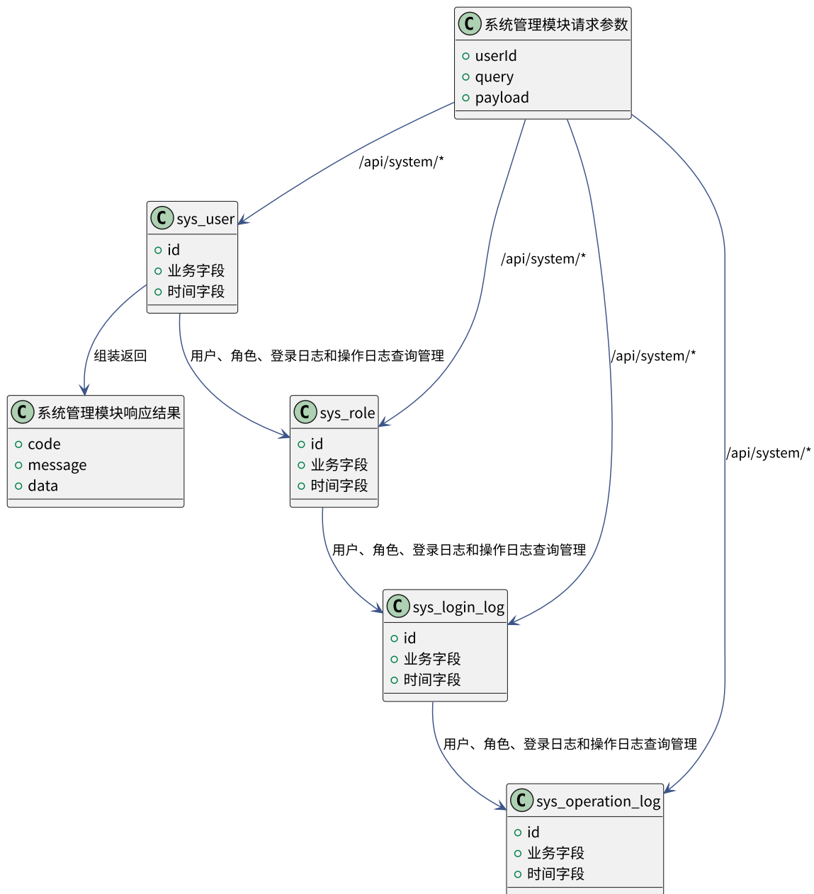
图 5-40 系统管理模块数据关系 UML 图
