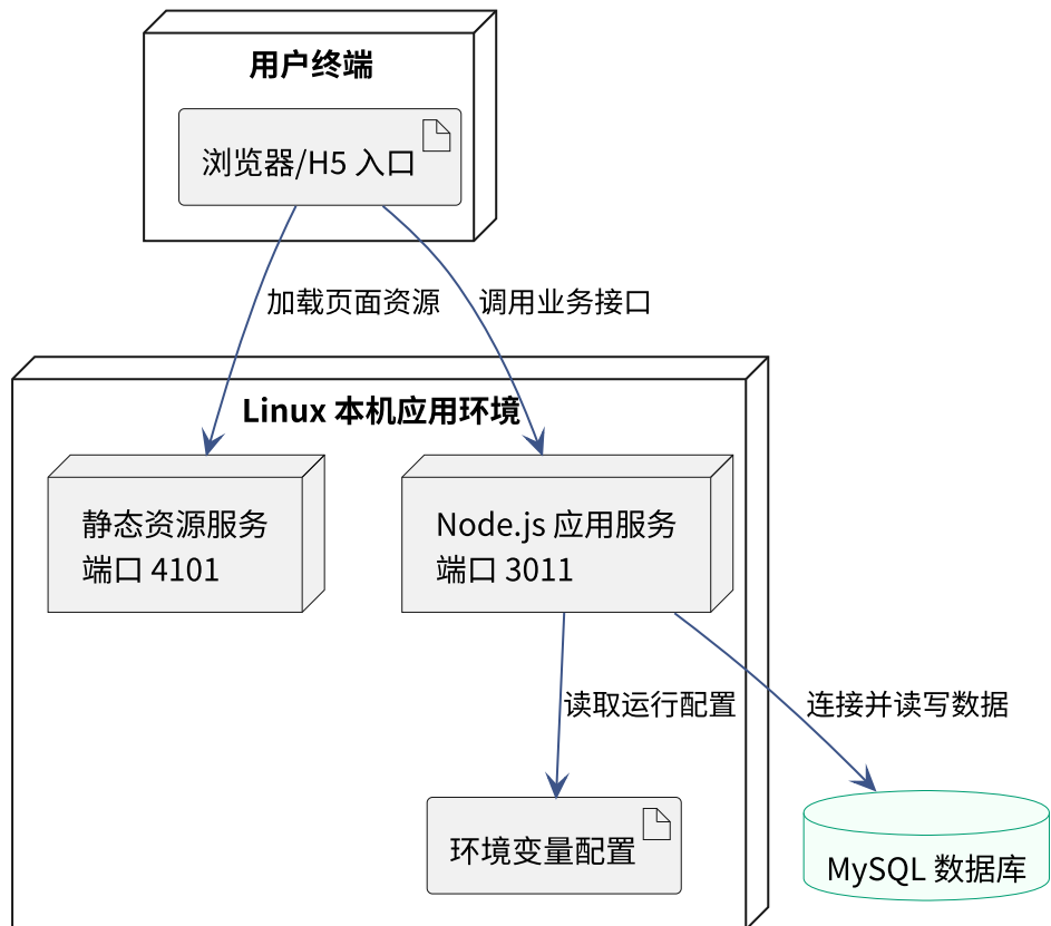
图 5-2 部署 UML 图
