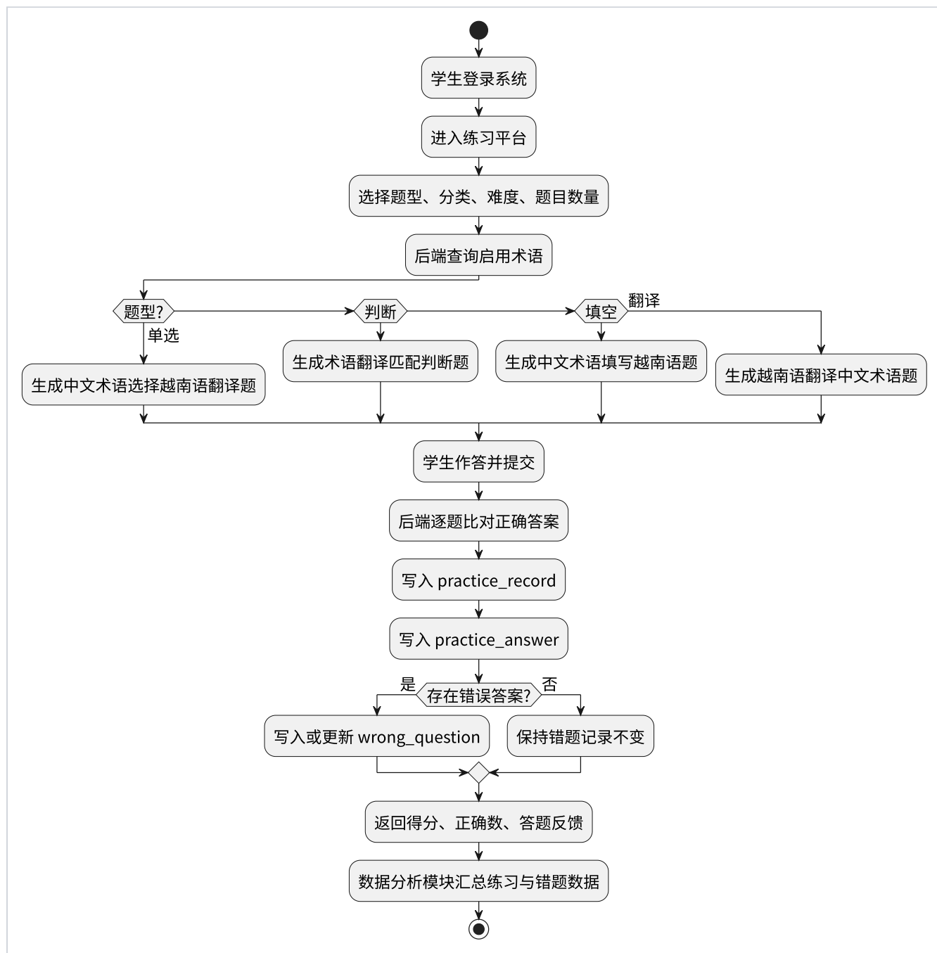
图4 练习业务流程图
