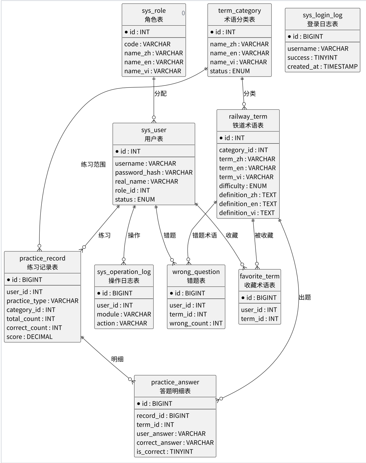
图5 数据库 ER 图
