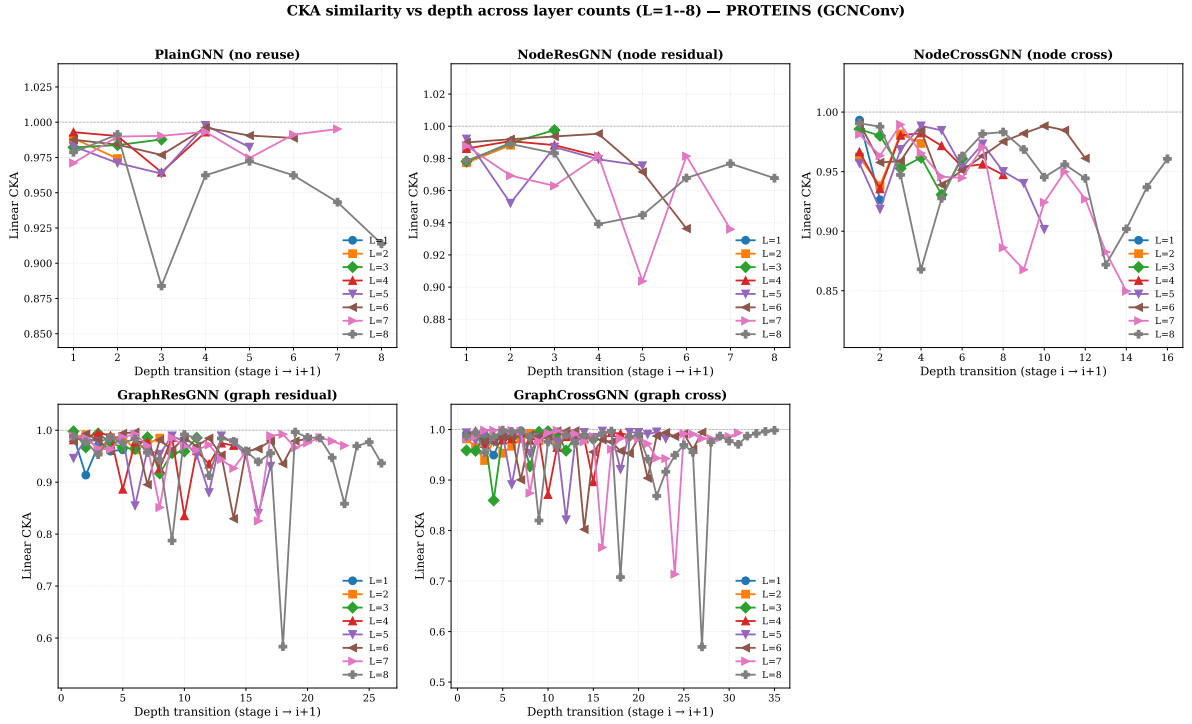
图 6: L = 1 到 L = 8 各层数下相邻深度阶段之间的 CKA 相似性。每个子图展示一个模型, 曲线对应不同层数。CKA 越高表示跨深度的表示连续性越强。
