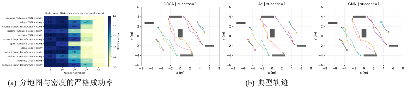
Fig. 5. (a) 各地图族与不同群体规模下的严格无碰撞成功率； random 与 narrow 布局在高密度下最具挑战性。(b) 典型轨迹，通信边以瞬时连线的形式绘制于半径内的机器人之间。
