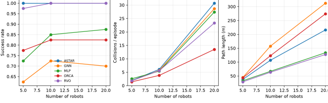
Fig. 2. 冻结的 600 回合评估中各方法与不同机器人规模的聚合对比。经典控制器在成功率与路径长度上占优，学习策略以完成率换取更低的单步开销。
