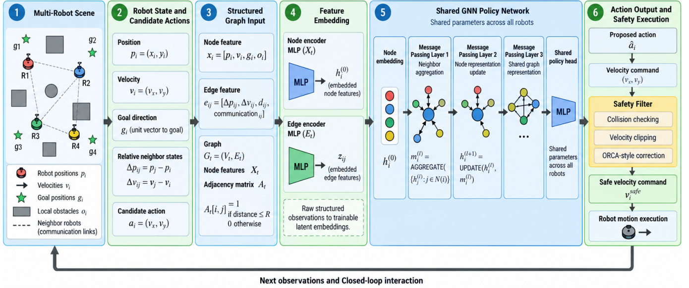
Fig. 1. 多机器人导航流程：机器人场景与状态、结构化图输入、特征嵌入、共享 GNN 推理，以及动作输出与可选安全过滤。执行后的运动反馈形成观测-动作闭环。
