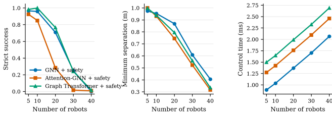
Fig. 4. 安全过滤下不同机器人规模的严格无碰撞成功率、最小间距与平均控制时间。机器人数量超过 20 后，无碰撞成功率下降。
