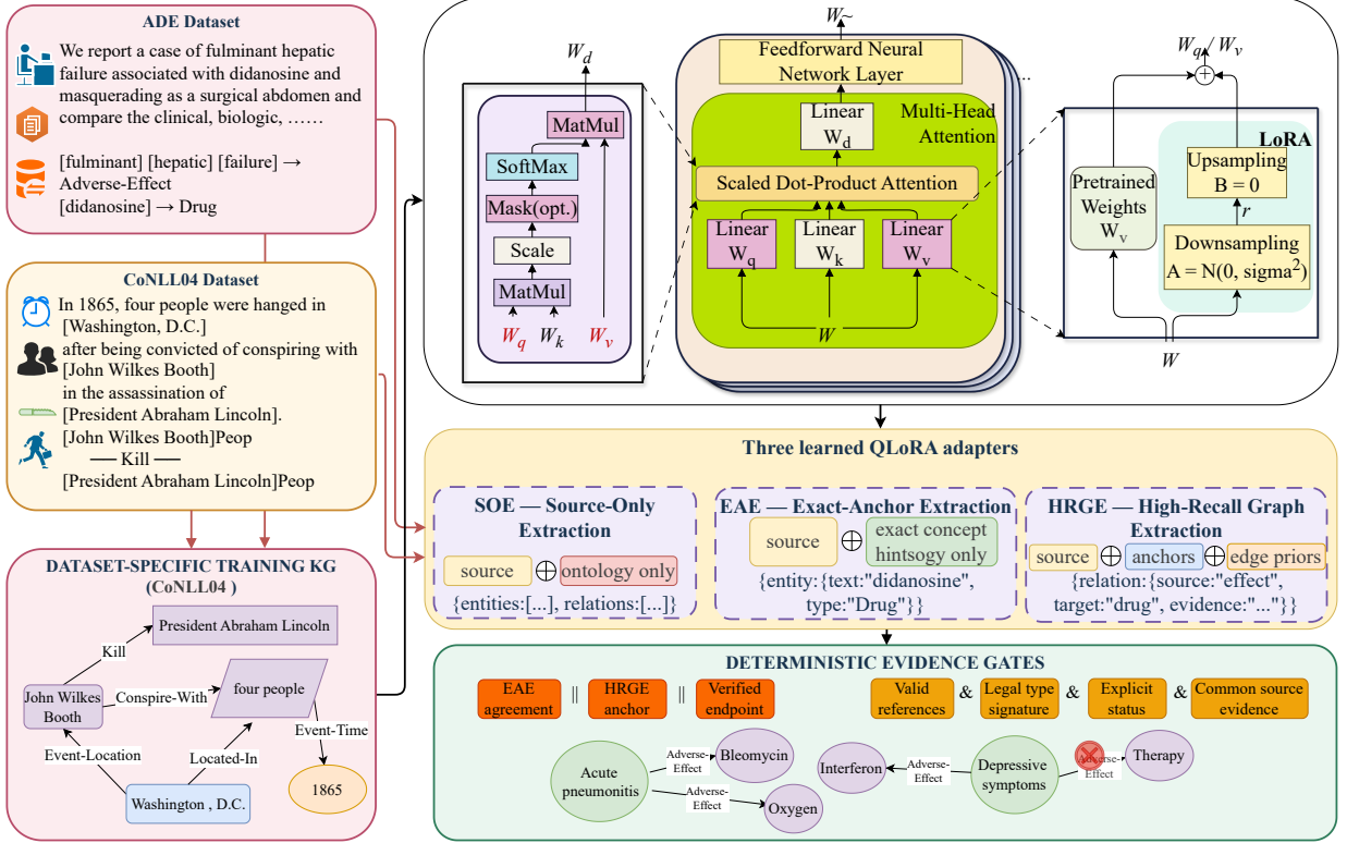
图 1: 本文采用的详细方法流程图。图中保留 ADE 与 CoNLL04 输入、数据集专属训练知识图谱、Transformer 注意力模块、SOE/EAE/HRGE 三个 QLoRA 适配器分支，以及由一致性、锚点、端点、关系有效性和共同证据组成的确定性证据门控。
