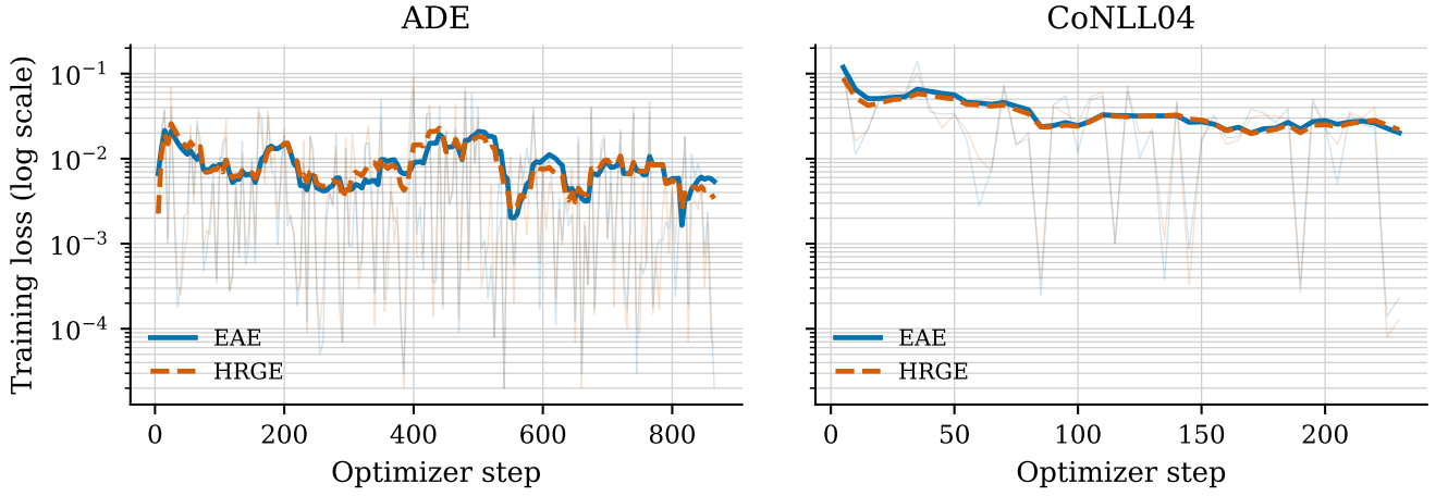
图 4: EAE 与 HRGE 适配器的训练损失。浅色线为每五个优化步采样的原始观测，强调曲线为十个观测点的尾随均值；对数尺度保留原始波动。
