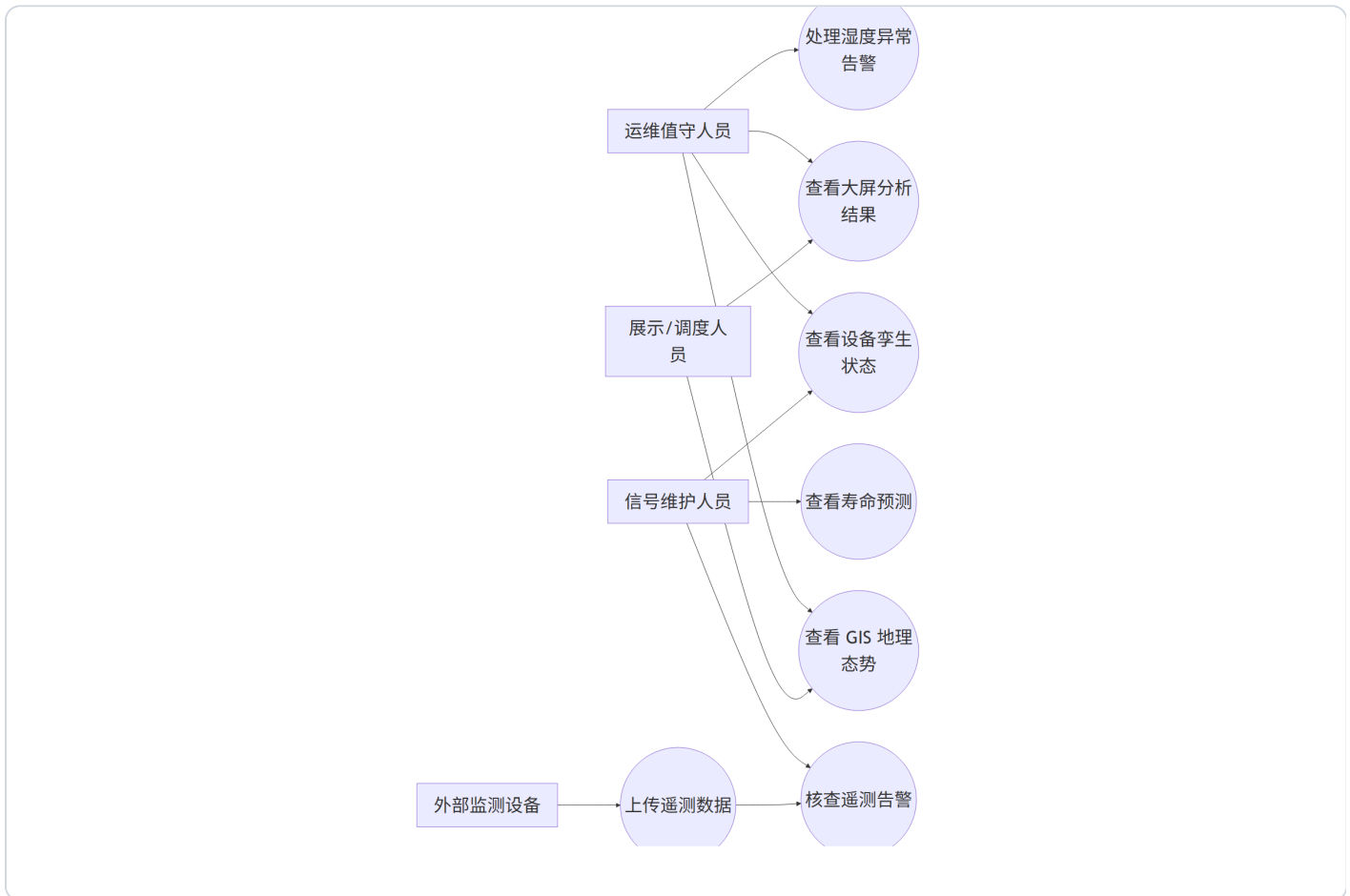
图 3-1 系统用例图
