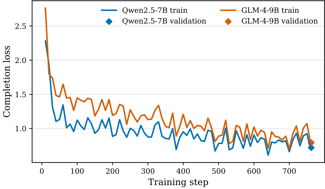
图 4: Qwen2.5-7B 和 GLM-4-9B 的仅答案监督 QLoRA 优化过程。曲线表示日志记录的训练损失；菱形表示每个模型唯一的 epoch 末验证点。
