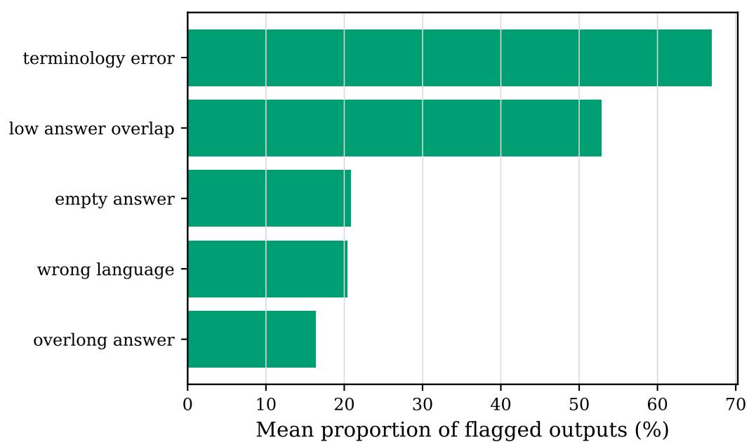
图 7: 独立双语问答及领域/翻译输出标记。柱形表示出现对应标记的模型条件/任务组内比例的均值，不是合并样本后的发生率。各标记不互斥；RAG 检索遗漏与引用缺失另见正文。
