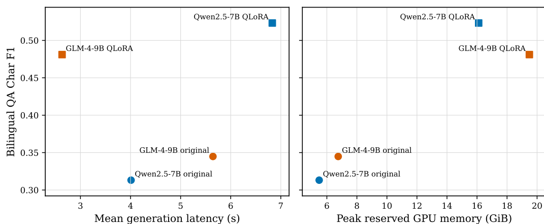
图 6: Qwen2.5/GLM 原始与 QLoRA 四种条件下, 独立问答双语平均字符级 F1 与生成时延、峰值预留显存 (GiB) 的关系。左图为平均生成时延; 右图为 PyTorch 预留显存。质量与资源在不同负载上测量。
