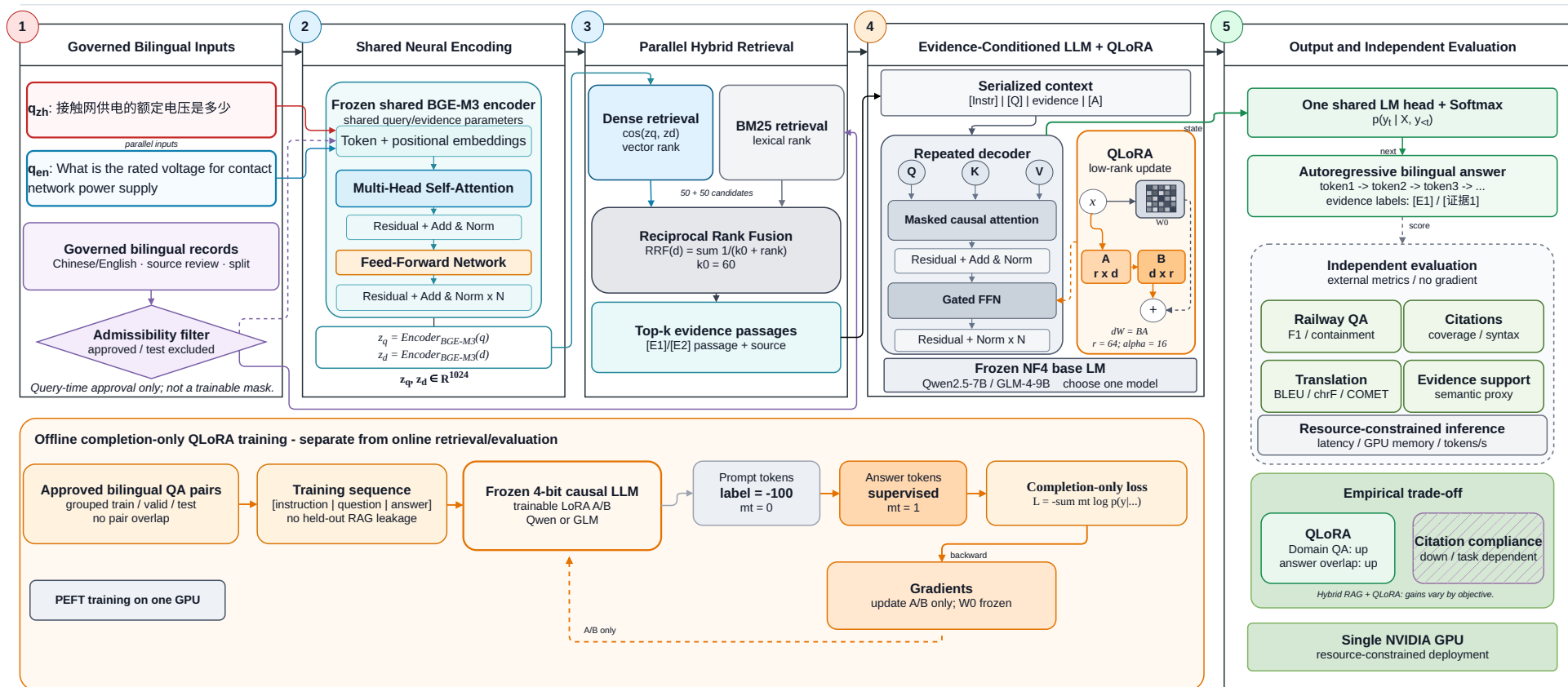
图 1: 双语铁路问答的混合检索与 QLoRA 架构。阶段 1–5 连接受治理输入、冻结的 BGE-M3 编码、BM25/密集检索排名融合、证据条件化生成及独立评估。下方分支展示基础权重冻结、仅答案监督的离线适配器训练；检索与评估不参与梯度更新。权衡标注为依赖任务的实证结果概括，不代表必然收益。来源：作者绘制。
