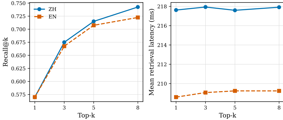
图 2: 最终证据截断点对融合检索的影响。召回率从 top-1 的 0.570 上升到 top-8 时中文的 0.743 与英文的 0.723，而平均检索时延保持在约 218 ms 与 209 ms，因为上游候选池固定为每个检索器 50 个段落。因此，提高融合截断点可以在不显著改变检索时间的情况下改善证据覆盖。来源：作者自制。
