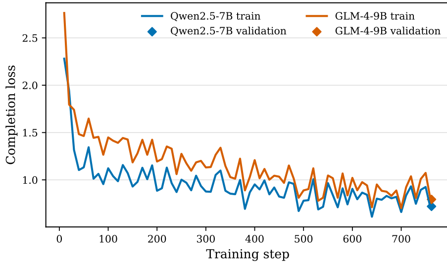
图 3: 单轮 completion-only QLoRA 优化。两个模型的训练损失都迅速下降随后趋于平缓；菱形标记轮末验证测量值，二者都贴近最终训练区间。Qwen2.5-7B 在两条曲线上都低于 GLM-4-9B，与其更强的留出结果一致。曲线支持在资源限制内成功完成优化，但不构成更长训练计划或重复随机种子下的结论。来源：作者自制。
