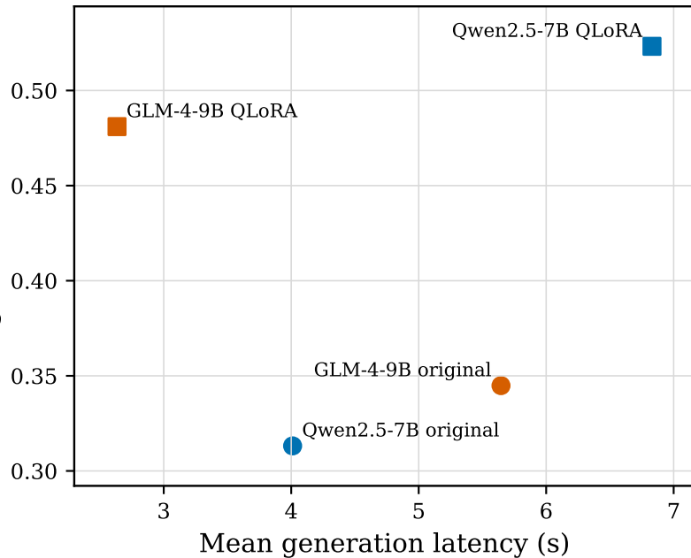
Bilingual QA Char F1
