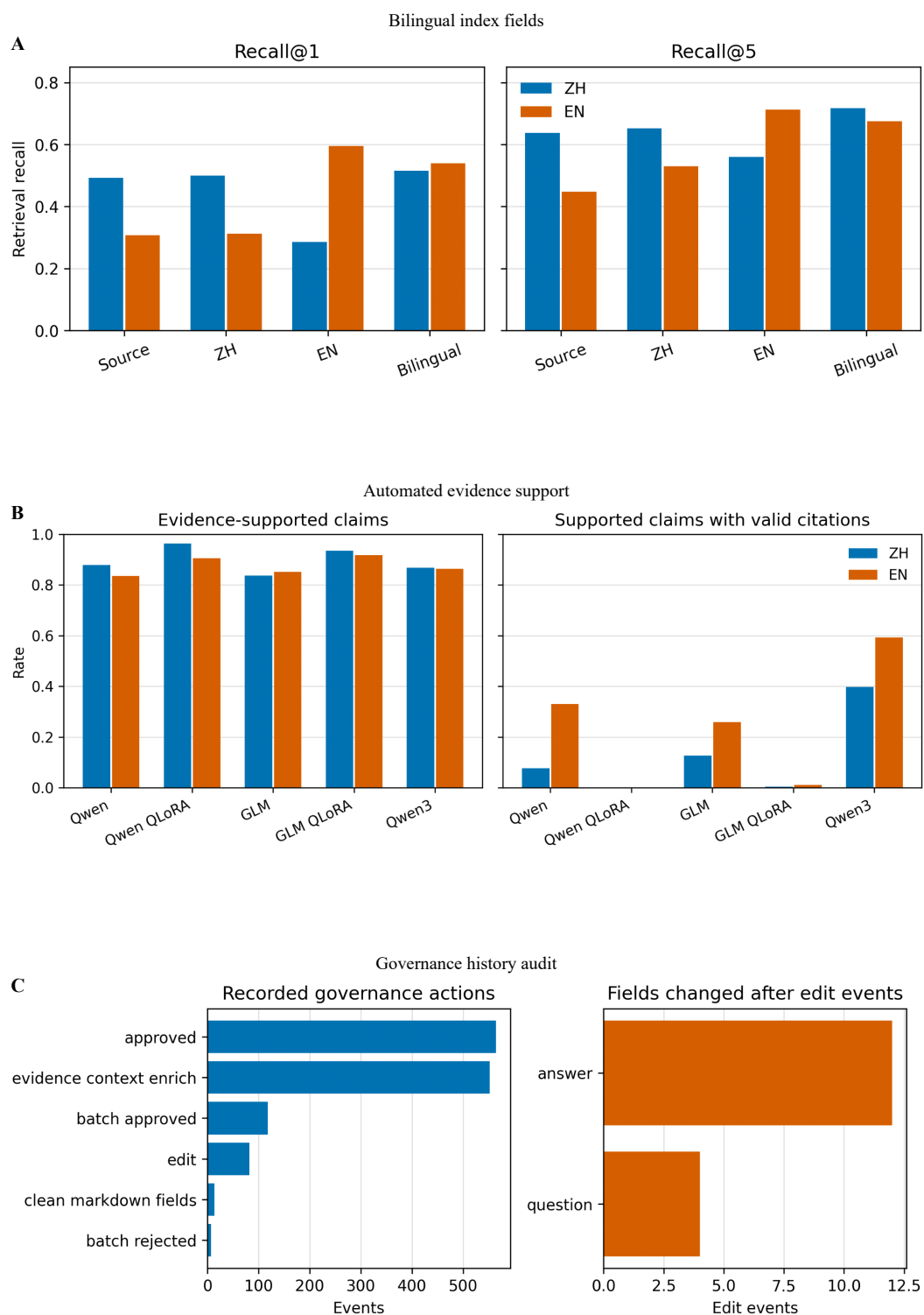
图 7: 三个验证层次。A 面板比较不同索引字段, B 面板比较检索证据与明确引用证据的语义支持, C 面板审计不可变审核事件和修改前状态快照。三个面板分别表达检索均衡性、证据支持和治理可追溯性, 不合并为单一分数。
