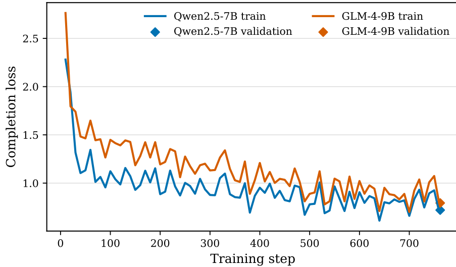
图 3: Qwen2.5-7B 和 GLM-4-9B 的仅答案监督 QLoRA 优化过程。曲线表示日志记录的训练损失；菱形表示每个模型的 epoch 末验证点。
