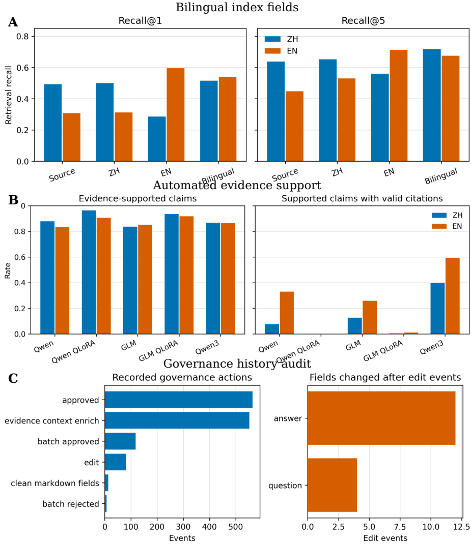
图 5: 三个验证层次。A 面板比较仅源字段、语言专用字段和双语字段索引；双语字段在两种语言之间取得更好的均衡结果，而语言专用字段可能在单一语言上更强。B 面板比较检索证据与明确引用证据的语义支持，说明相关证据访问与可见引用是不同属性。C 面板审计不可变审核事件和修改前状态快照，说明治理动作与变更字段能够保持可追溯。三个面板分别表达检索均衡性、证据支持和治理可追溯性，不合并为单一分数。“—”表示该指标不按语言分别统计。
