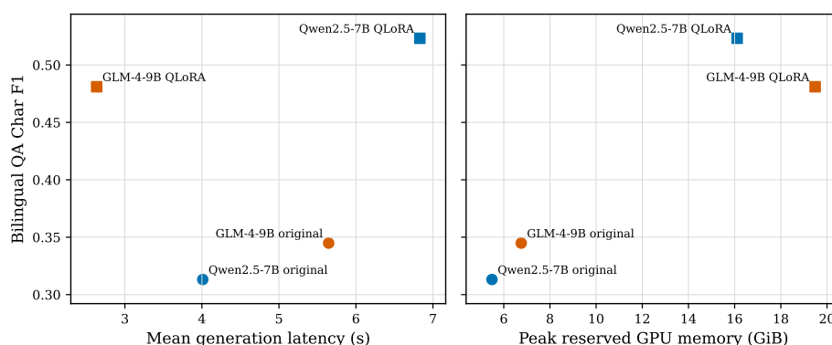
图 4: Qwen2.5/GLM 原始与 QLoRA 四种条件下，独立问答双语平均字符级 F1 与生成时延、峰值预留显存 (GiB) 的关系。左图为平均生成时延；右图为 PyTorch 预留显存。质量与资源在不同负载上测量。
