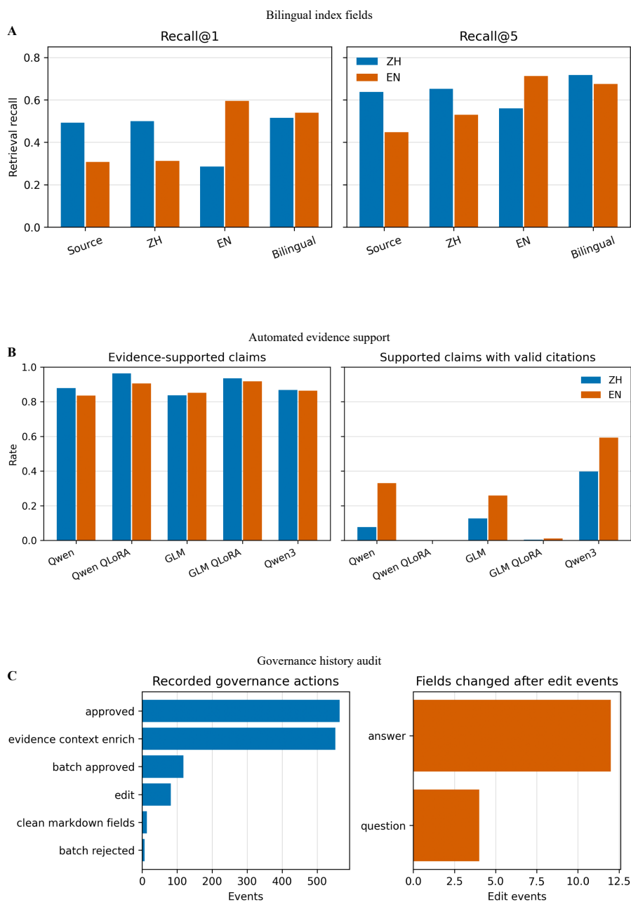
图 5: 三个验证层次。A 面板比较不同索引字段，B 面板比较检索证据与明确引用证据的语义支持，C 面板审计不可变审核事件和修改前状态快照。三个面板分别表达检索均衡性、证据支持和治理可追溯性，不合并为单一分数。
