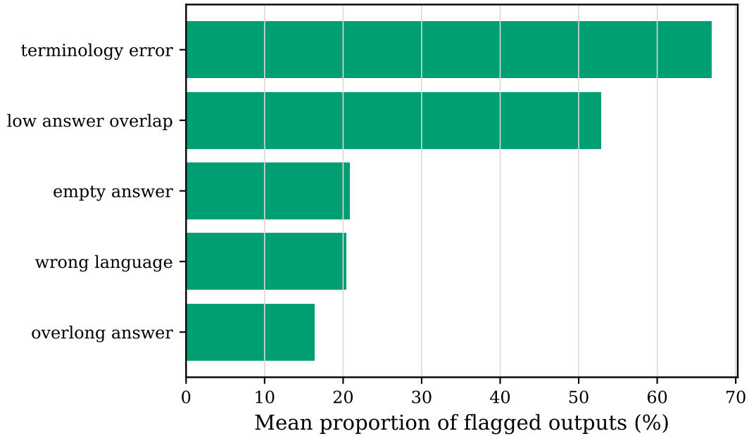
图 7: 各生成器和检索条件下自动标记输出错误的平均比例。
