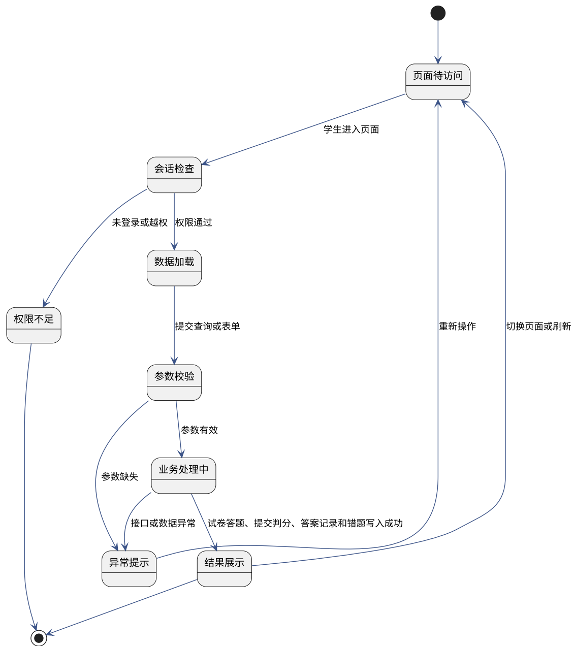
面向马来西亚留学生的汉语练习平台在线答题模块状态图
