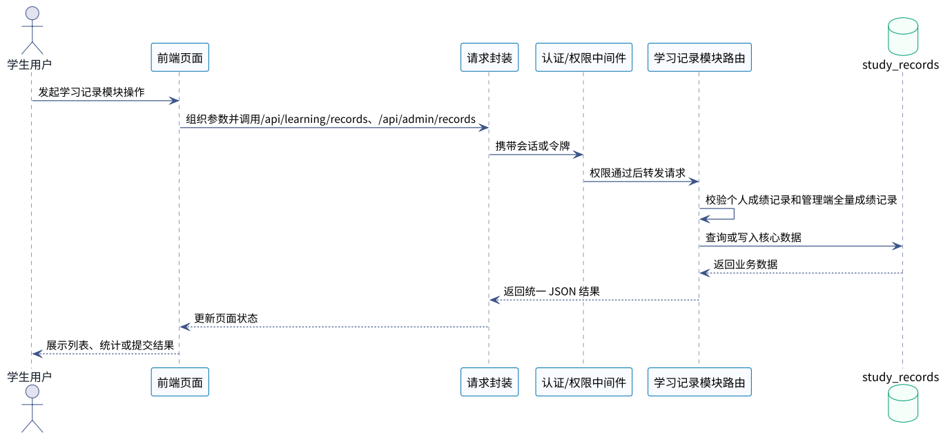
面向马来西亚留学生的汉语练习平台学习记录模块时序图
