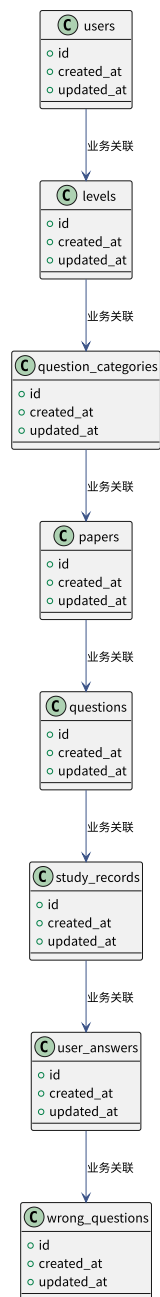
图 5-4 数据对象 UML 类图
