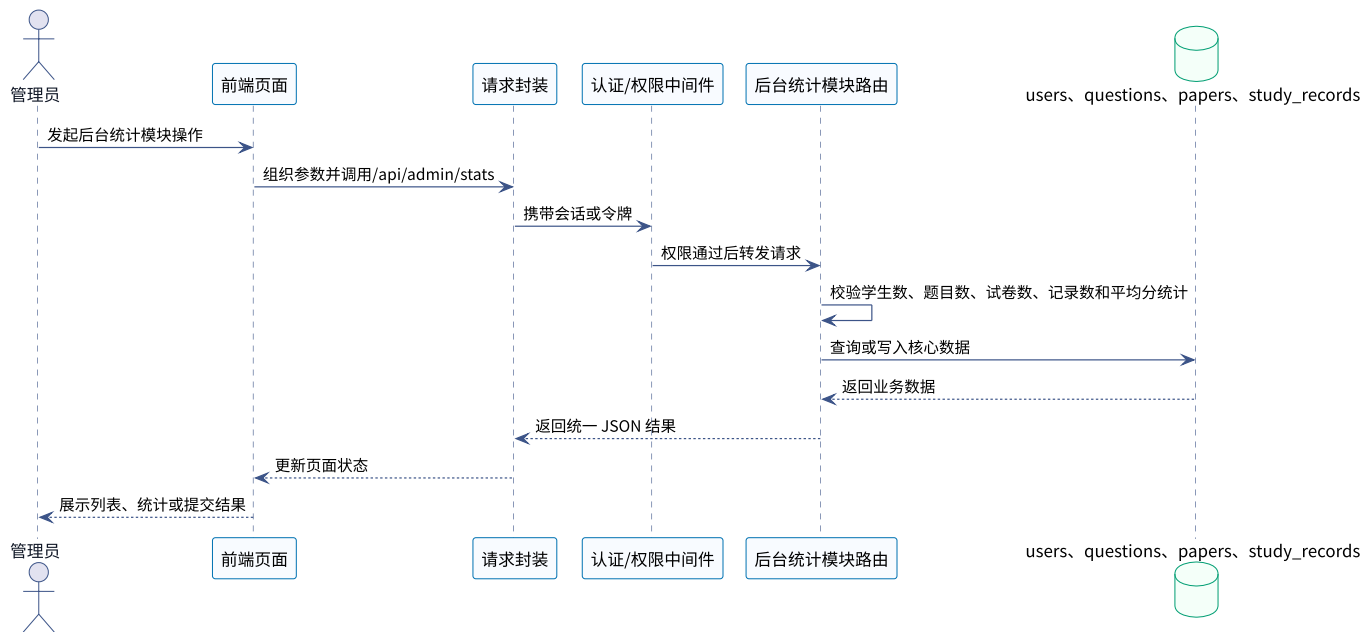
面向马来西亚留学生的汉语练习平台后台统计模块时序图
