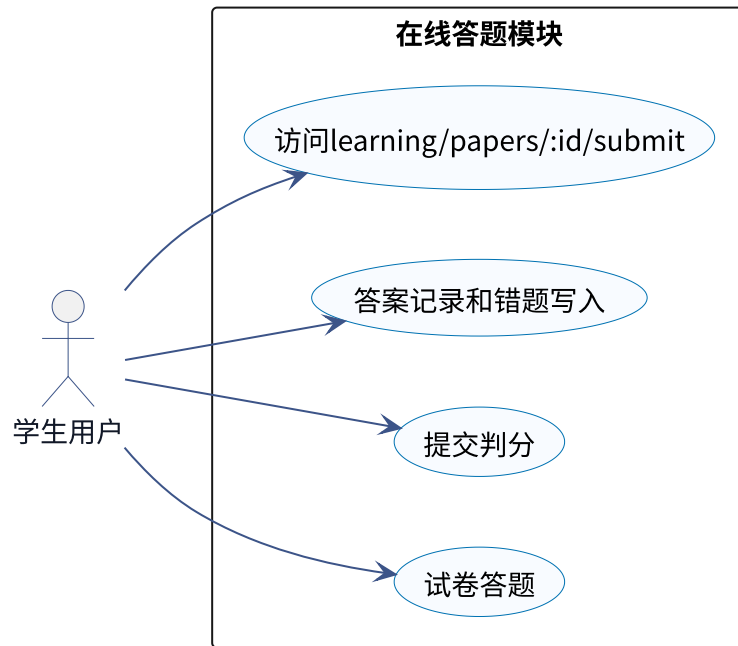
图 5-17 在线答题模块用例 UML 图
