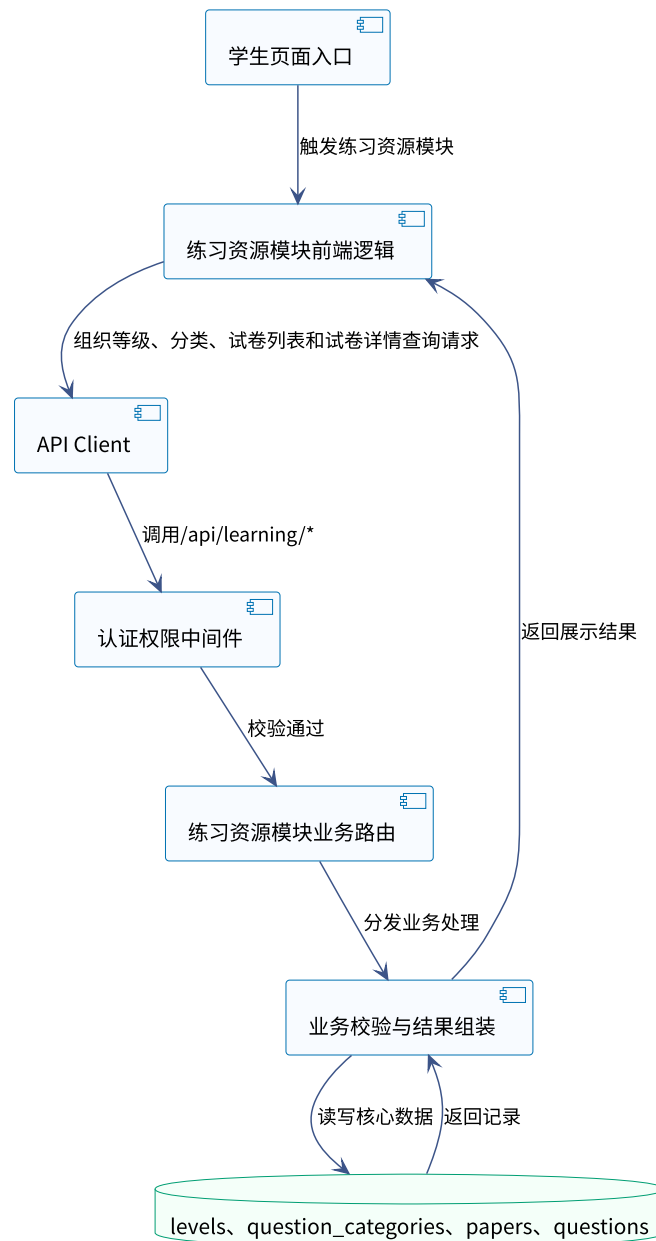
面向马来西亚留学生的汉语练习平台练习资源模块组件协作图
