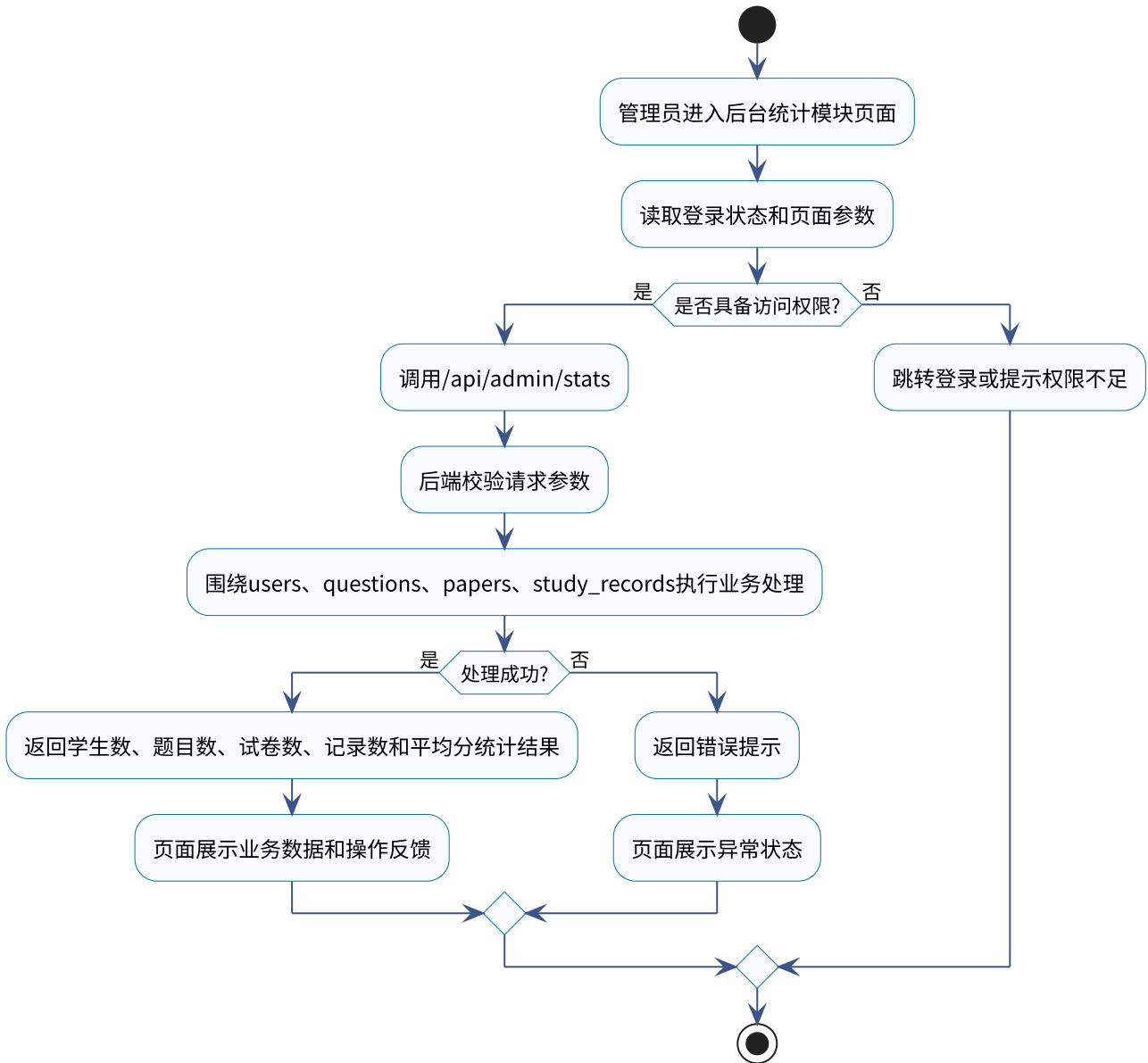
面向马来西亚留学生的汉语练习平台后台统计模块活动图
