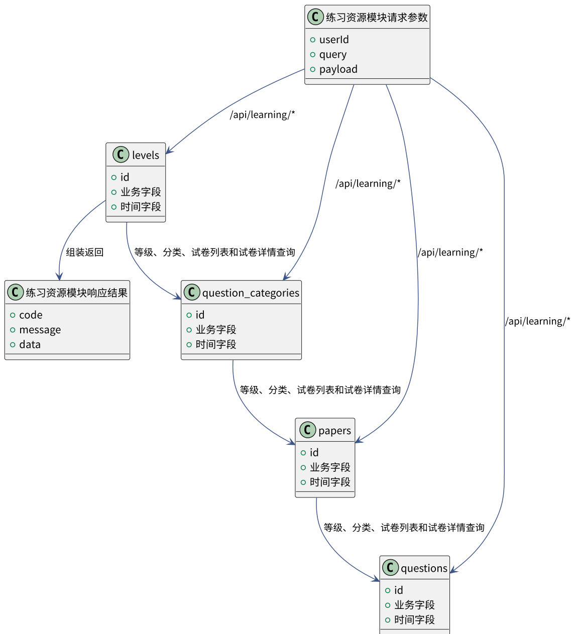
图 5-16 练习资源模块数据关系 UML 图
