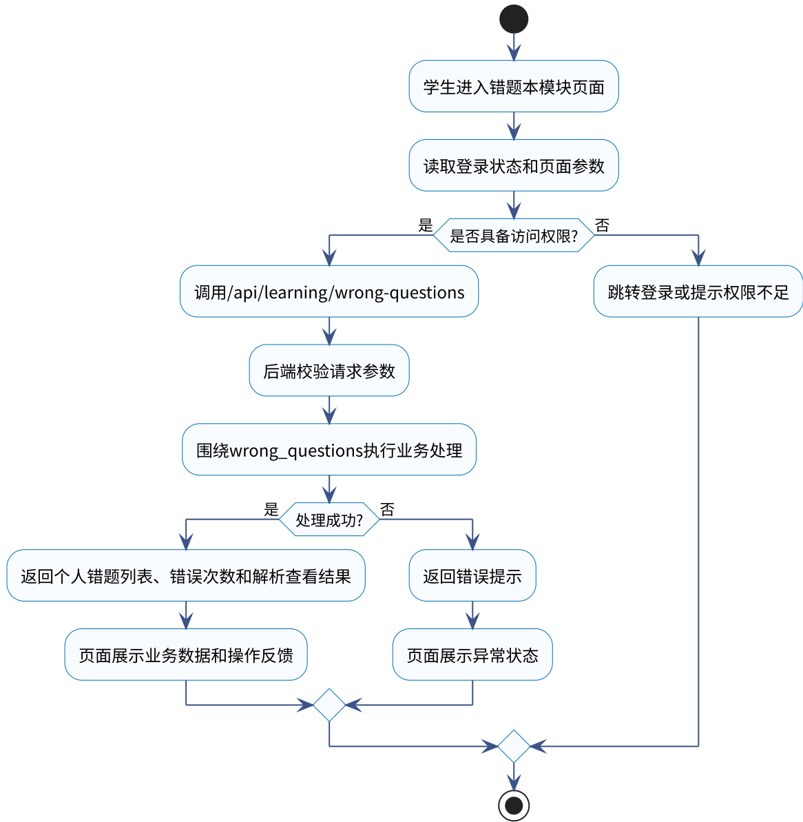
面向马来西亚留学生的汉语练习平台错题本模块活动图
