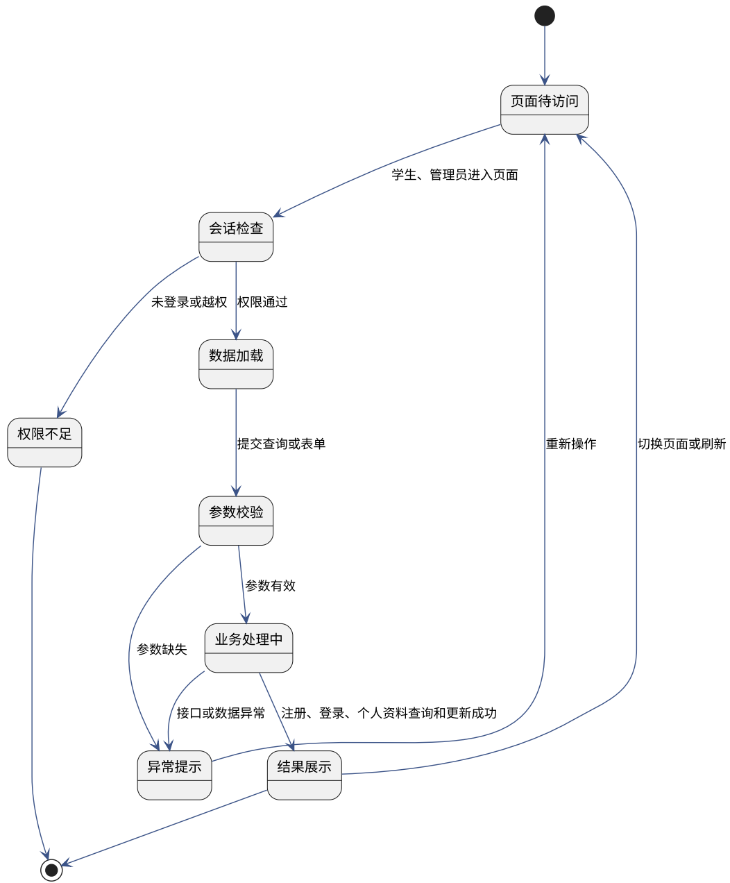
图 5-8 认证与资料模块状态 UML 图
