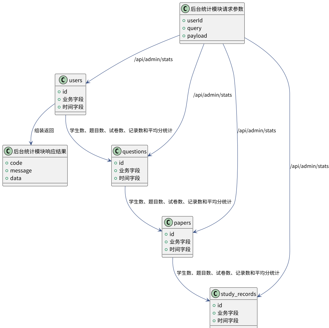
面向马来西亚留学生的汉语练习平台后台统计模块数据关系图
