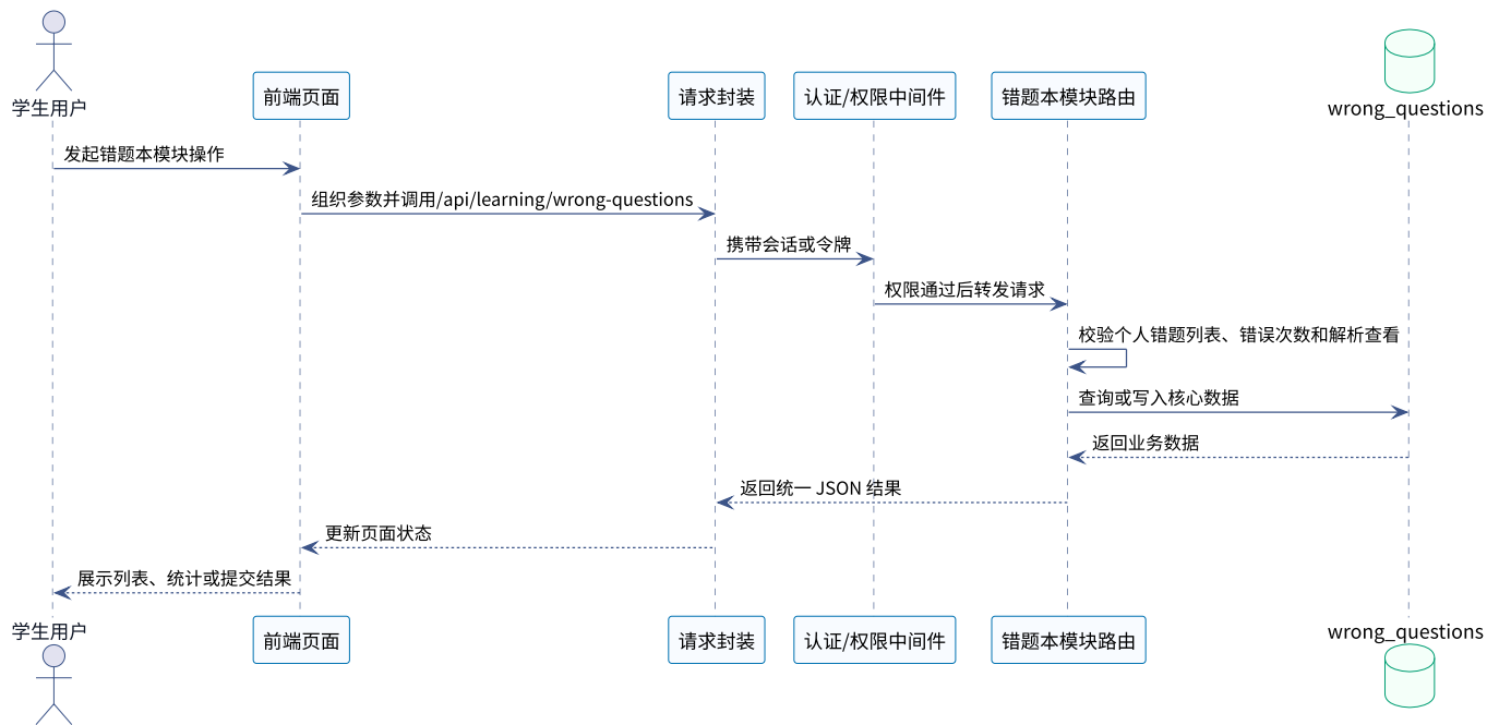
面向马来西亚留学生的汉语练习平台错题本模块时序图
