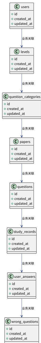
图 6-1 数据对象关系 UML 图
