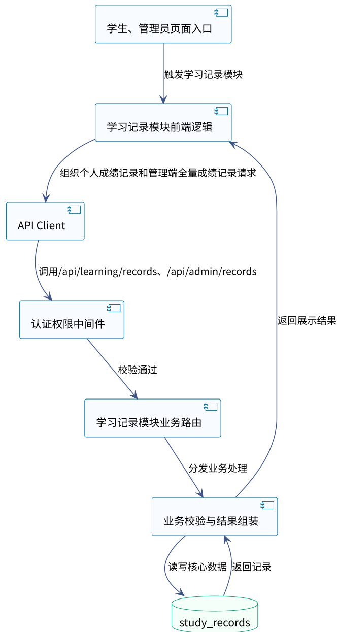
面向马来西亚留学生的汉语练习平台学习记录模块组件协作图
