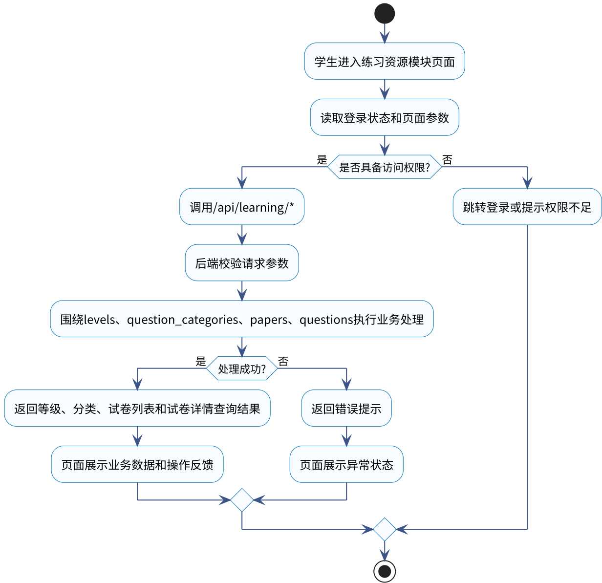
面向马来西亚留学生的汉语练习平台练习资源模块活动图
