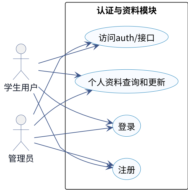
图 5-5 认证与资料模块用例 UML 图
