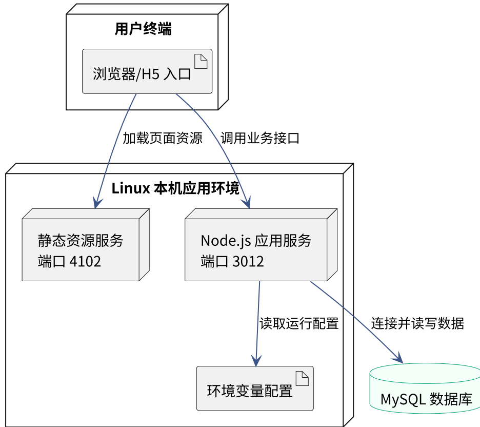
图 5-2 部署 UML 图
