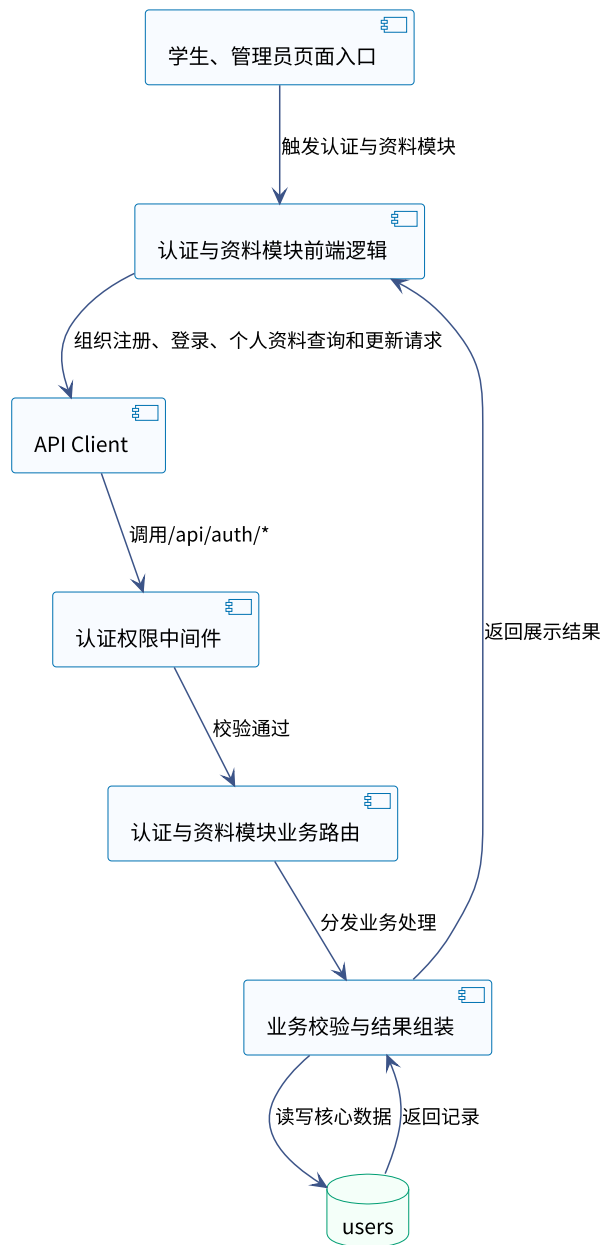
面向马来西亚留学生的汉语练习平台认证与资料模块组件协作图
