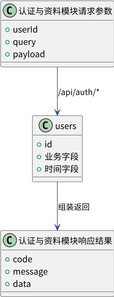
图 5-10 认证与资料模块数据关系 UML 图
