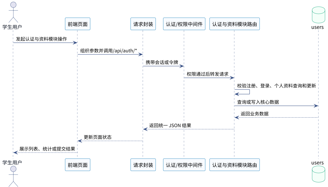
面向马来西亚留学生的汉语练习平台认证与资料模块时序图
