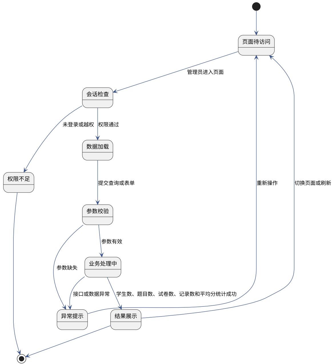
图 5-38 后台统计模块状态 UML 图
