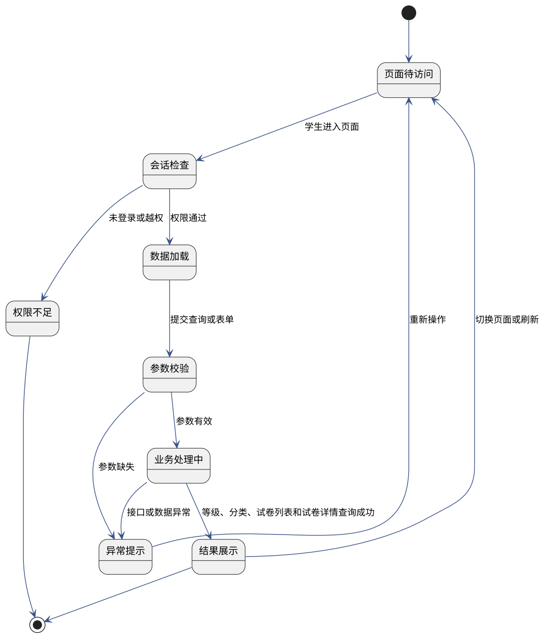
图 5-14 练习资源模块状态 UML 图
