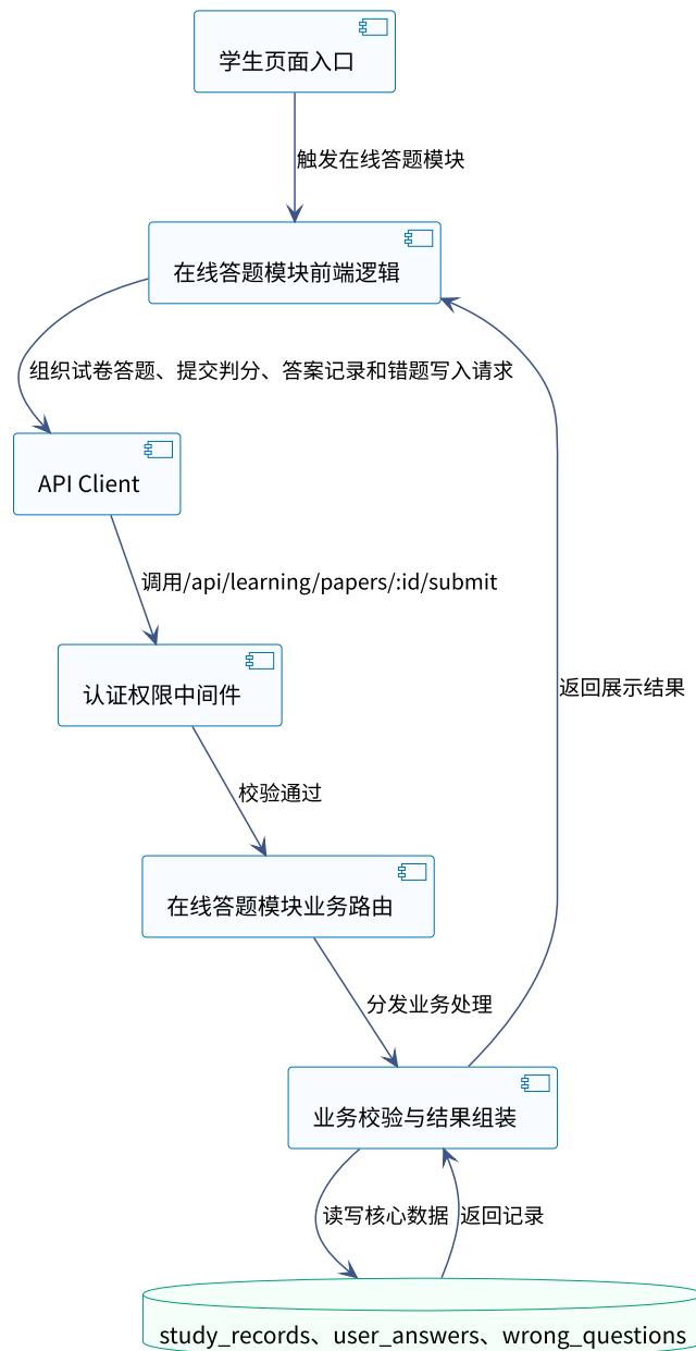
面向马来西亚留学生的汉语练习平台在线答题模块组件协作图
