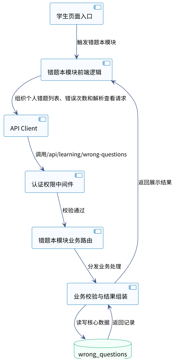
面向马来西亚留学生的汉语练习平台错题本模块组件协作图
