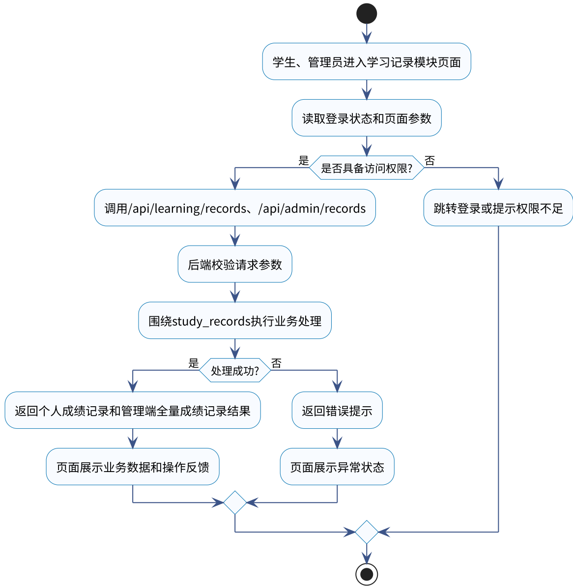
面向马来西亚留学生的汉语练习平台学习记录模块活动图
