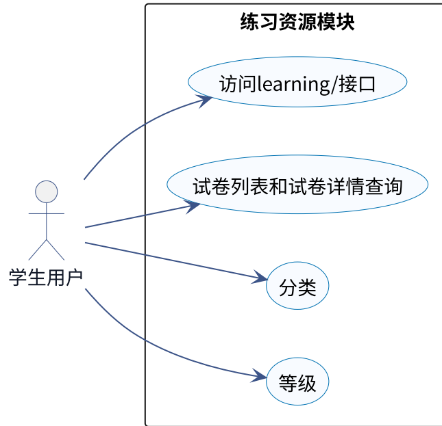
图 5-11 练习资源模块用例 UML 图
