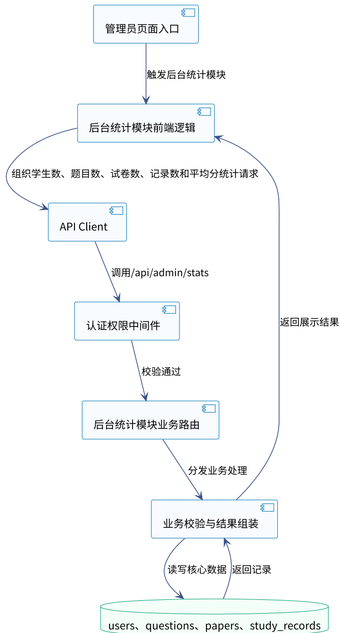
面向马来西亚留学生的汉语练习平台后台统计模块组件协作图
