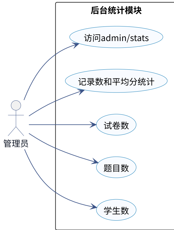
图 5-35 后台统计模块用例 UML 图
