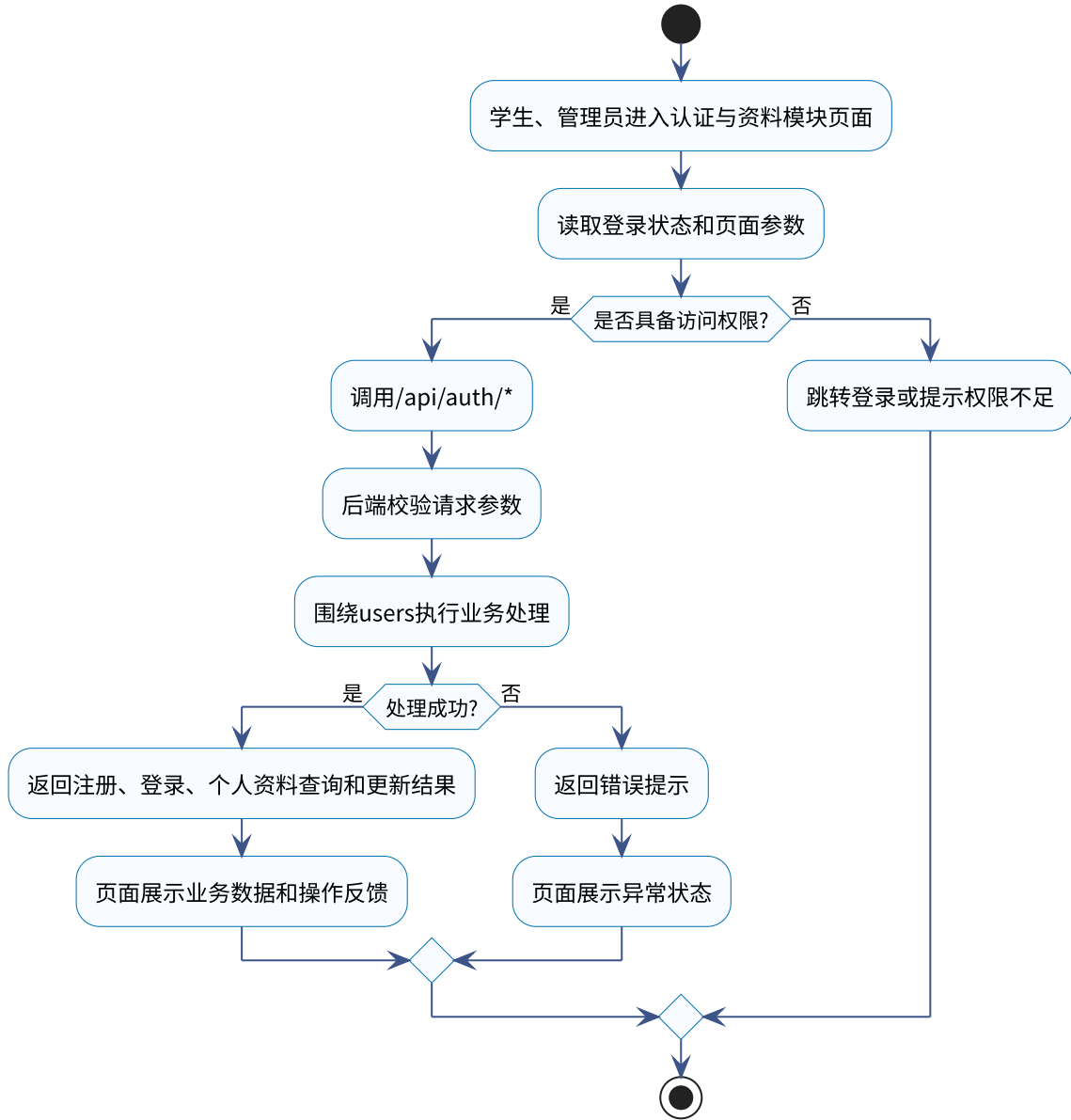
面向马来西亚留学生的汉语练习平台认证与资料模块活动图
