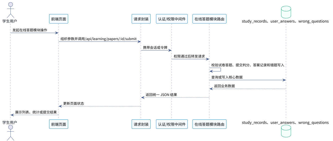
图 5-18 在线答题模块时序 UML 图
