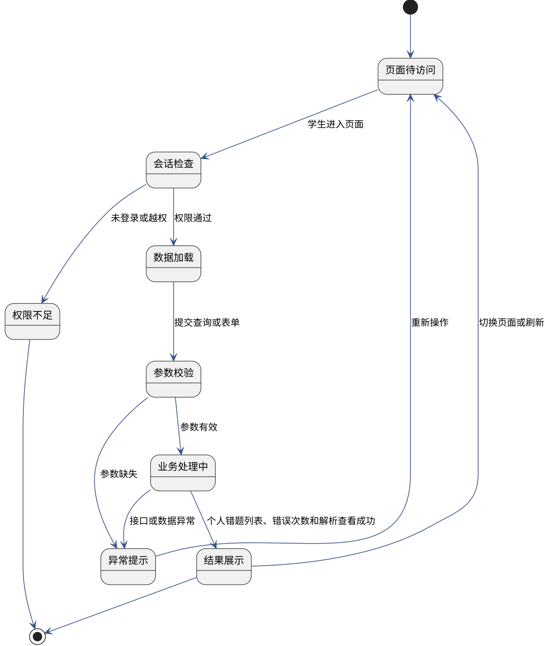
图 5-26 错题本模块状态 UML 图
