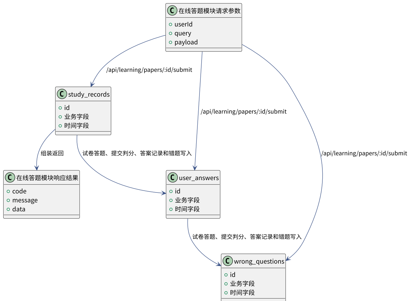
面向马来西亚留学生的汉语练习平台在线答题模块数据关系图
