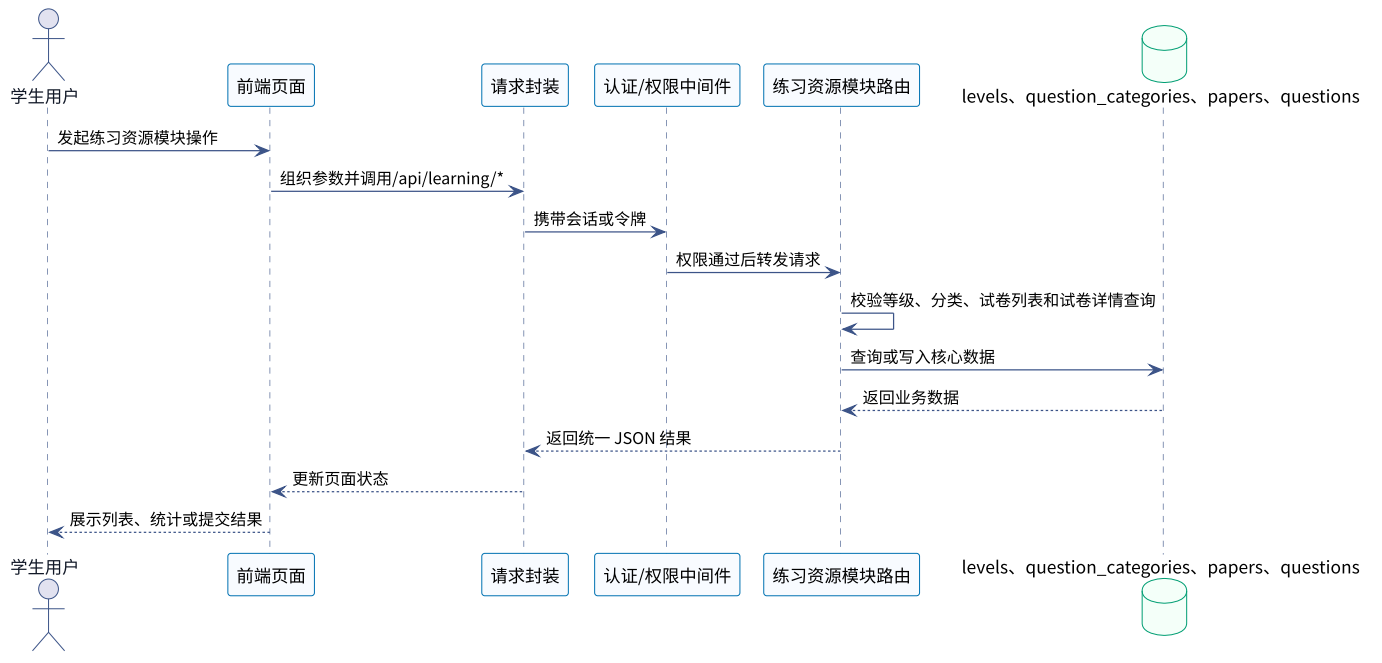
图 5-12 练习资源模块时序 UML 图
