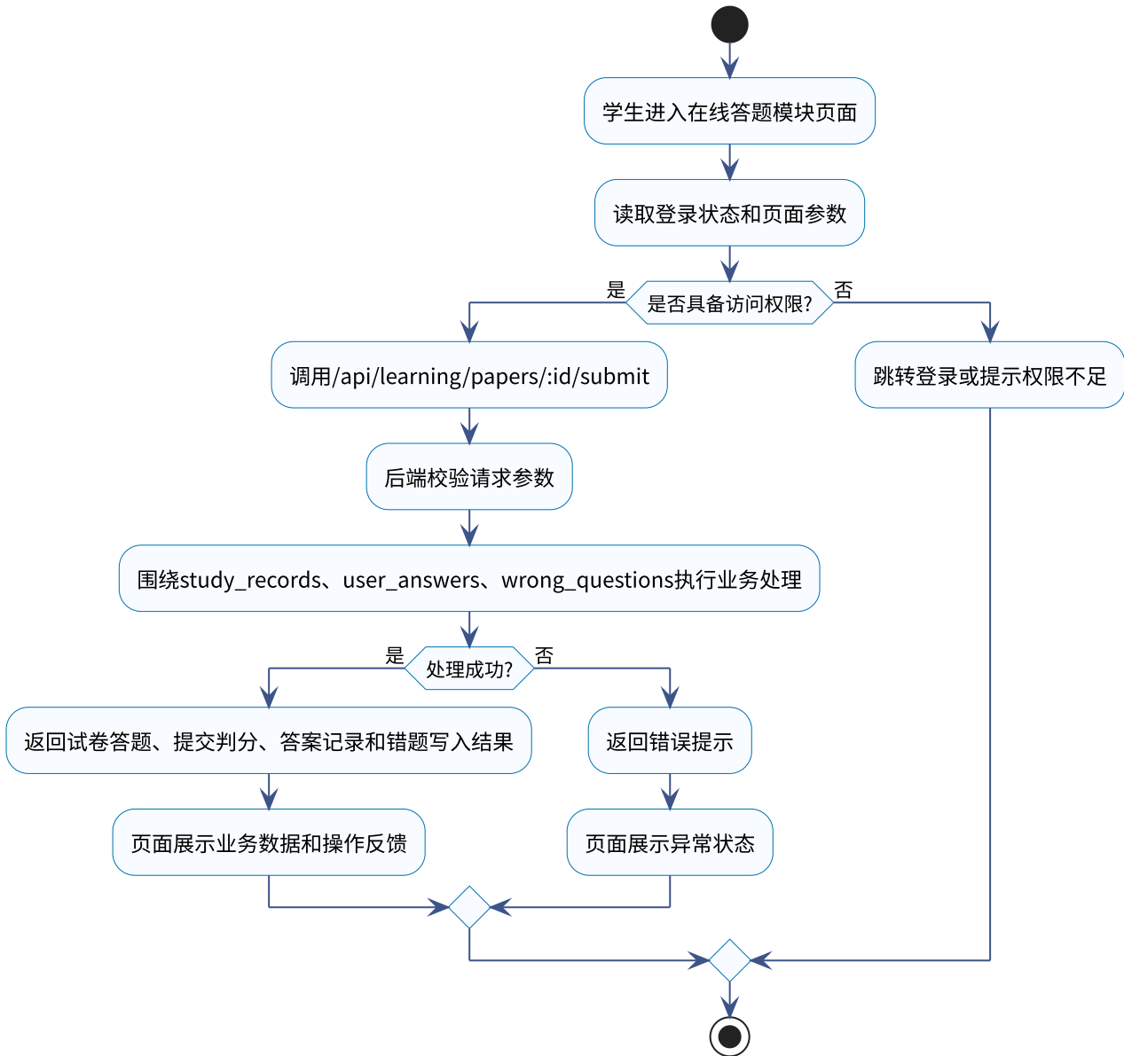
图 5-19 在线答题模块活动 UML 图
