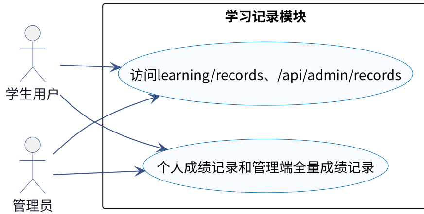
图 5-29 学习记录模块用例 UML 图
