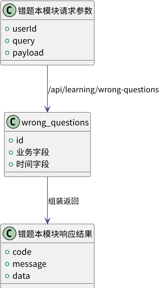
图 5-28 错题本模块数据关系 UML 图
