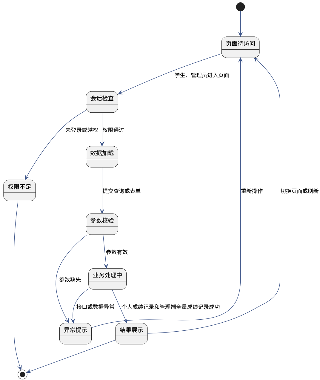
图 5-32 学习记录模块状态 UML 图
