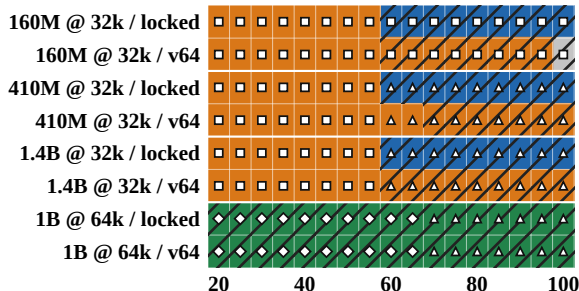
QA (2Wiki)
