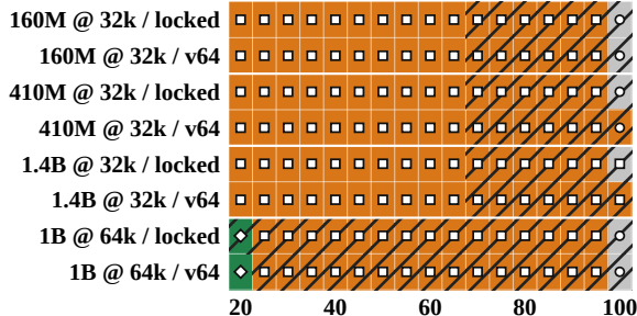
QA (2Wiki)
