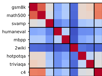
gemma3-4b
