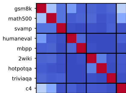
olmo3-7b
