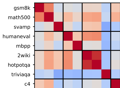
gemma3-1b
