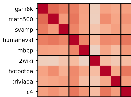
Qwen--Qwen3-1.7B
