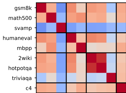
gemma3-270m
