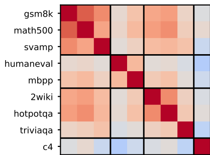
Qwen--Qwen3-4B
