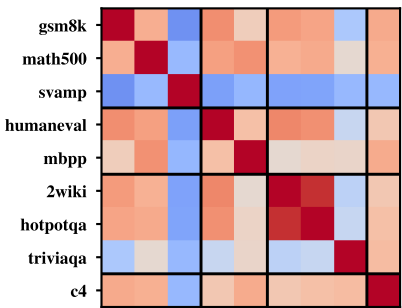
gemma3-270m
