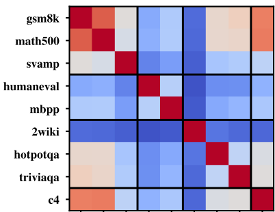
gemma3-4b
