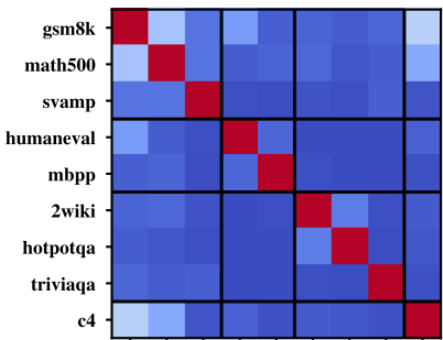
olmo3-7b
