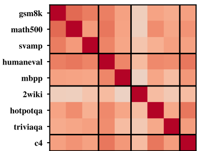
Qwen--Qwen3-1.7B
