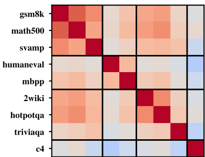
Qwen--Qwen3-4B
