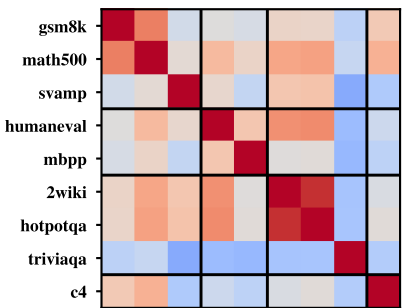
gemma3-1b
