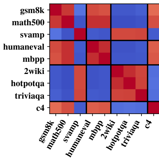
OLM03-7B
