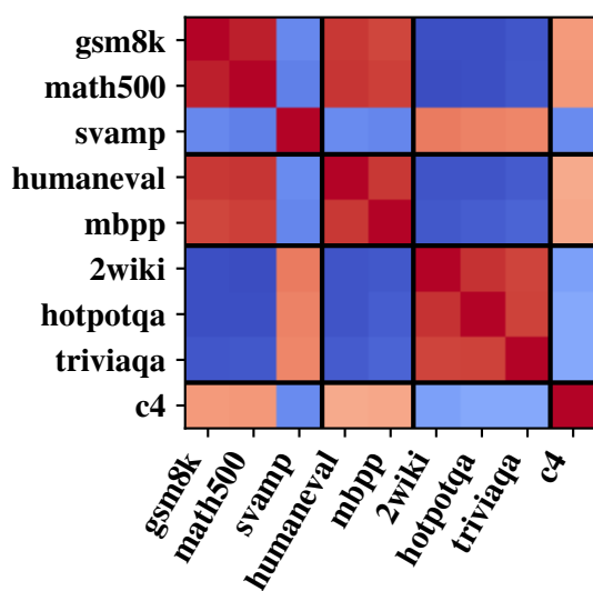
Gemma3-4B
