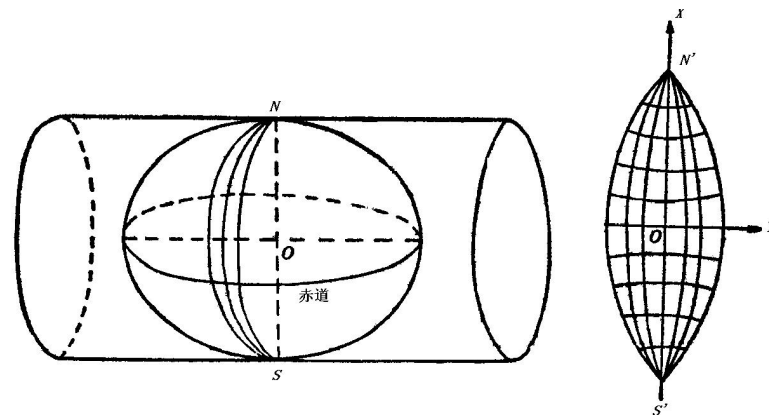
高斯—克吕格投影示意
