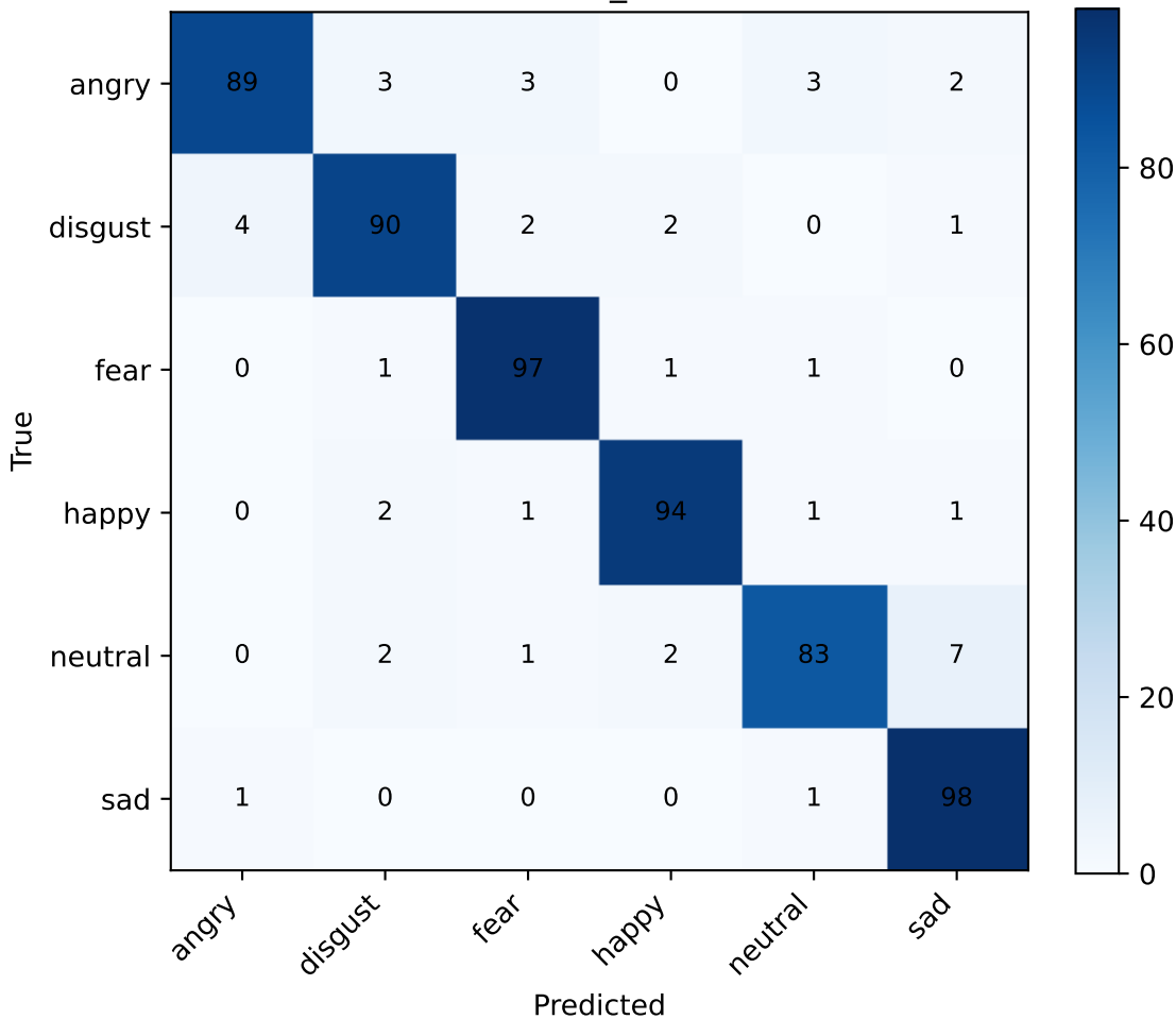
C-BESD_SelfAttn_frozen E1-02_s42
