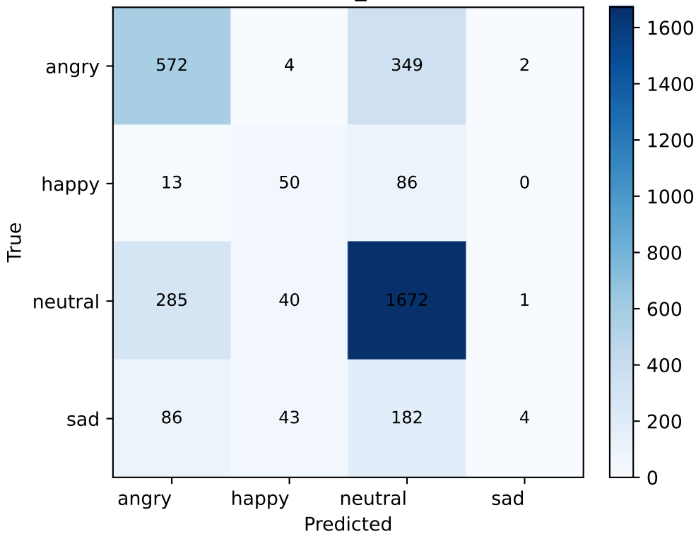
FAU_SelfAttn_frozen E1-05_s42
