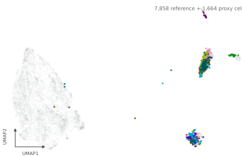
D. CellRank
