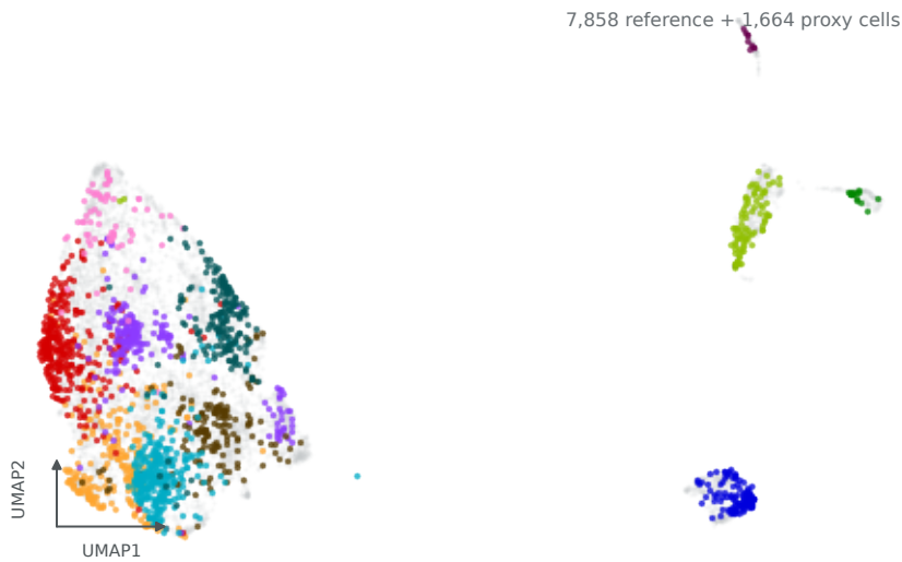
E. Leca-VC
