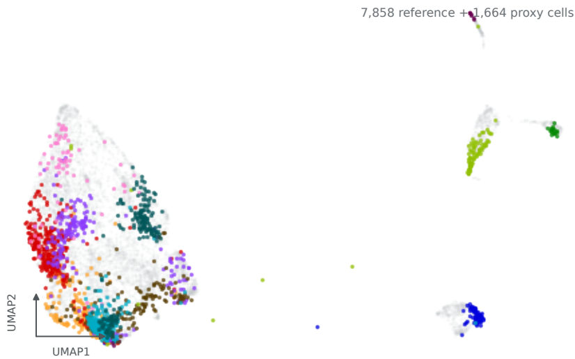
B. scGen
