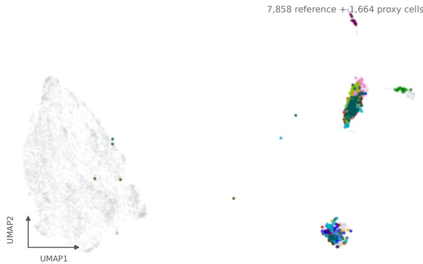
D. CellRank
