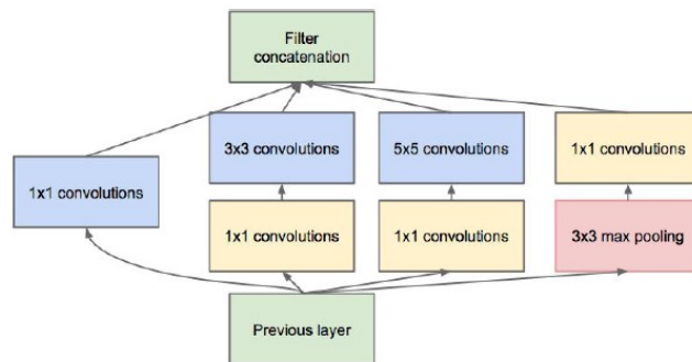
Inception module
