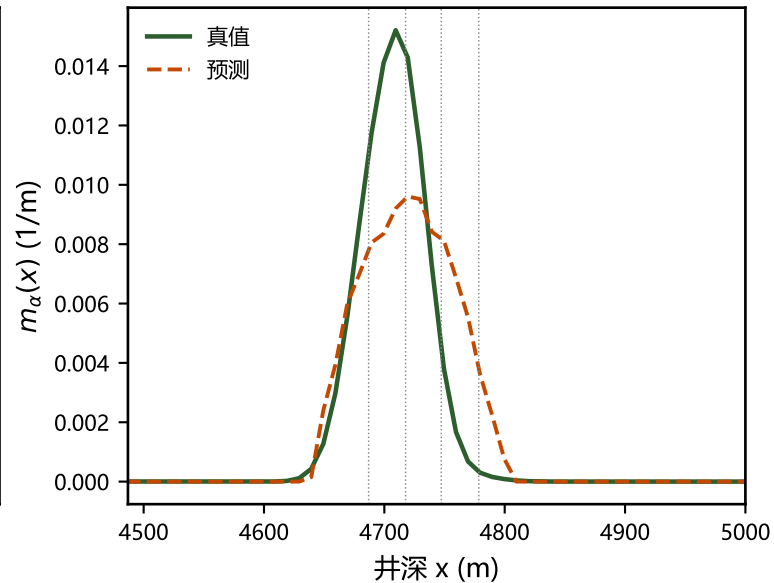
进液密度
