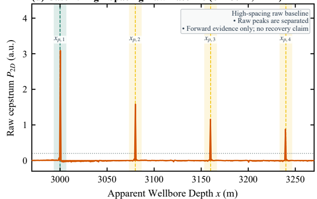
(d) Case 4: High-Spacing Raw Baseline ( S = 80 m, n = 4 )
