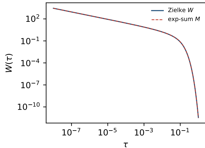
(d) memory-kernel fit
