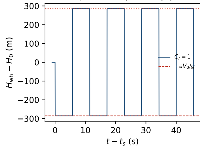
(a) Joukowski ideal pipe
