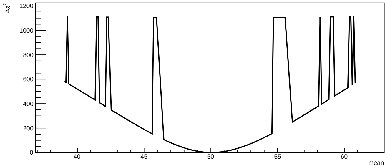
\chi^2 scan
