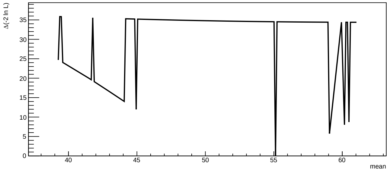
\chi^2 scan
