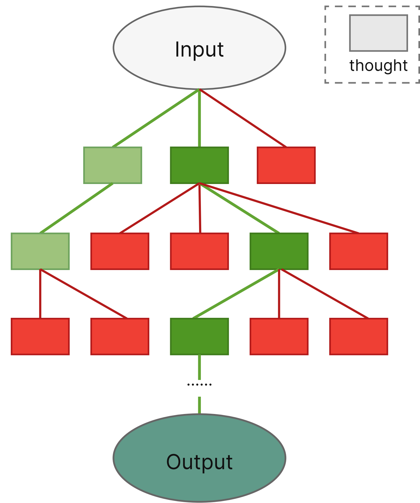
(d) Tree of Thoughts ( ToT )
